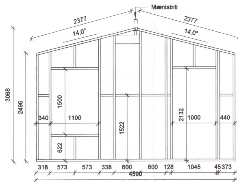
Suðurgafi 1 : 50
