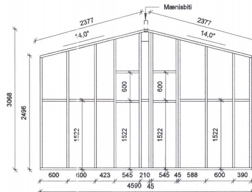
Norðurgafi 1 : 50
