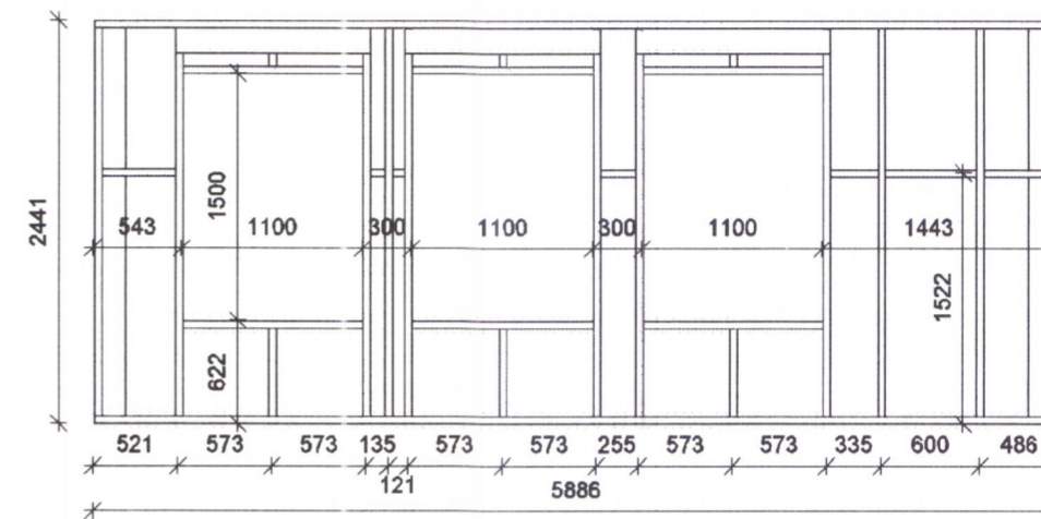
Austurhlið 1 : 50
