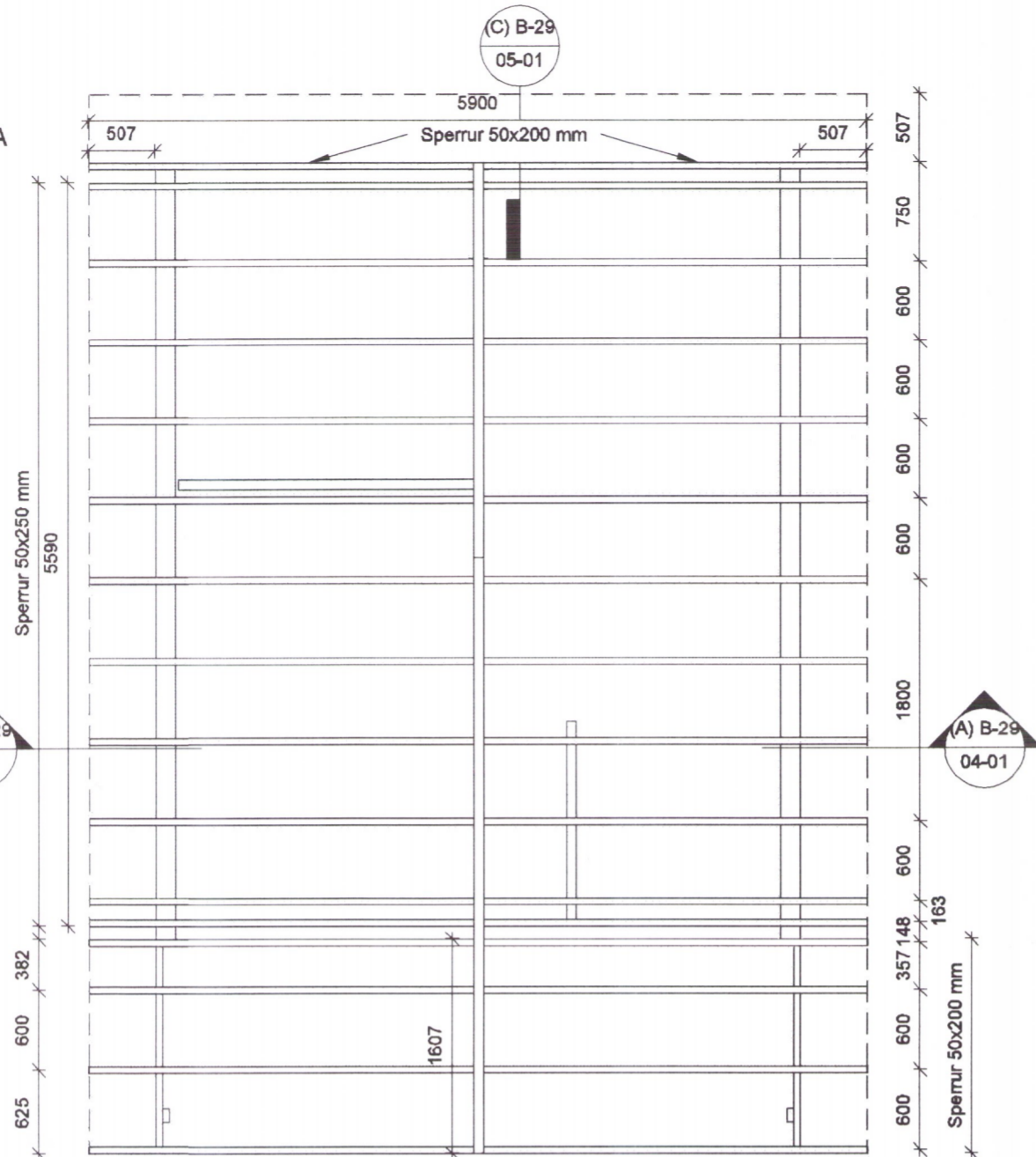
Sperruplan 1 : 50
