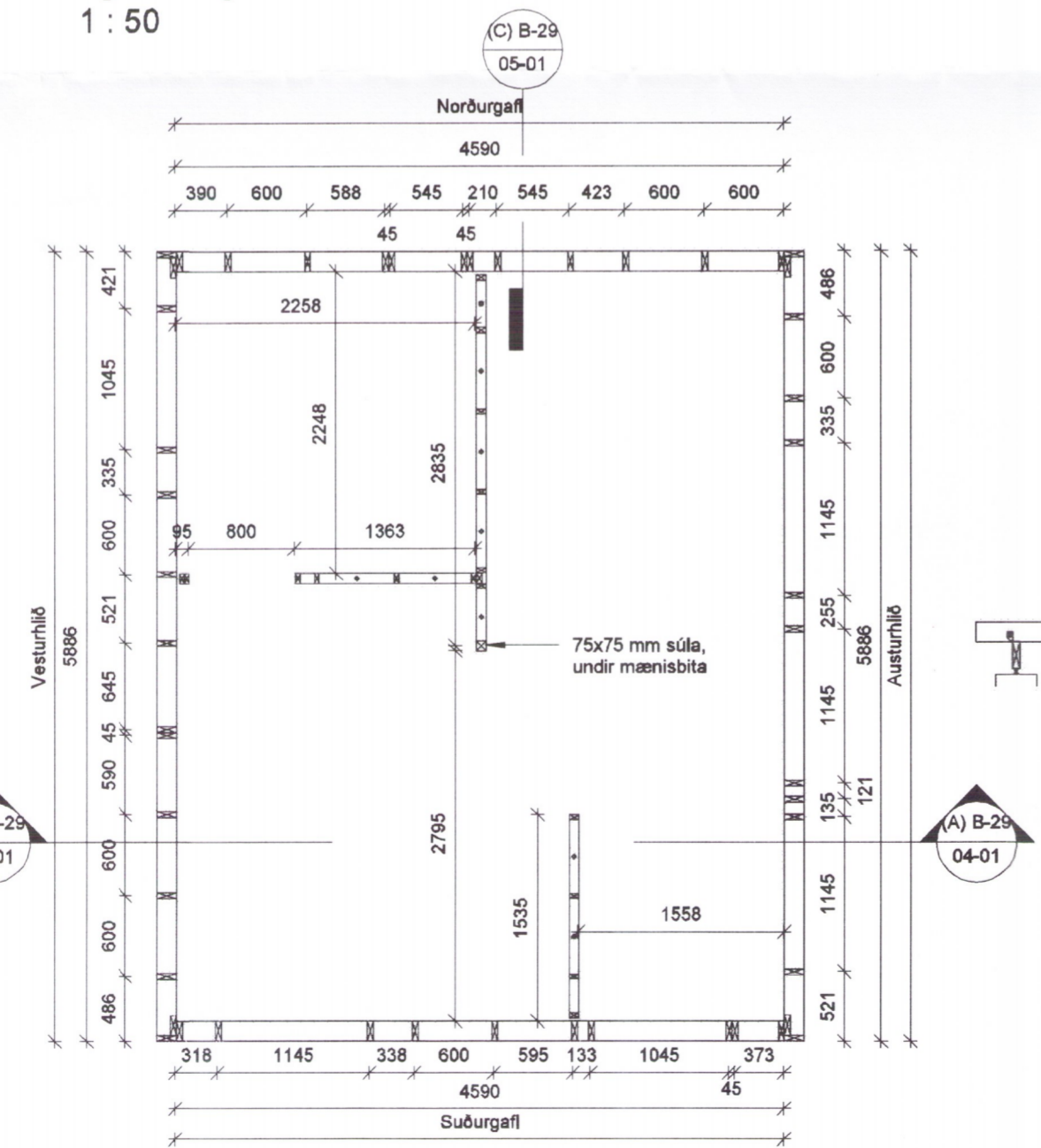
Sperruplan 1 : 50
