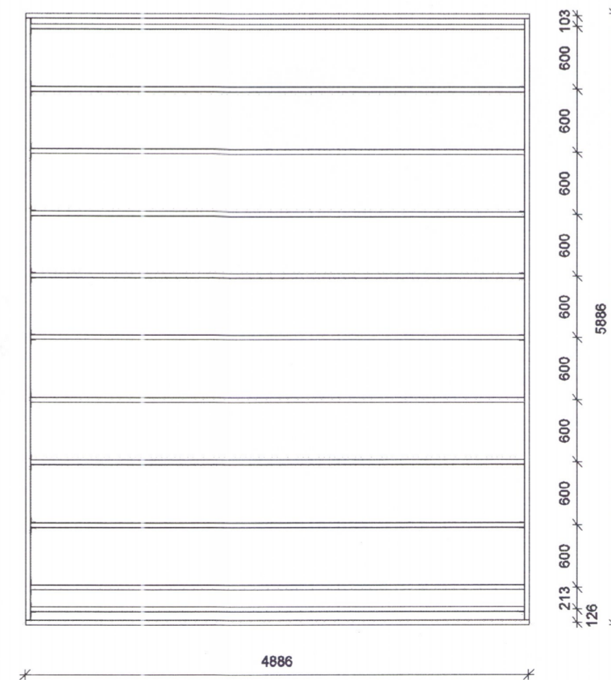
Gólfbitar 1 : 50
