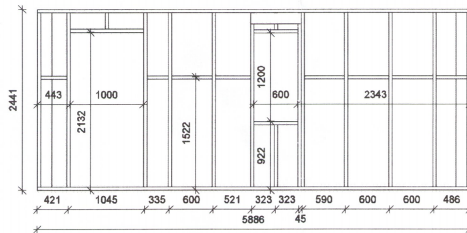
Vesturhlið 1 : 50
