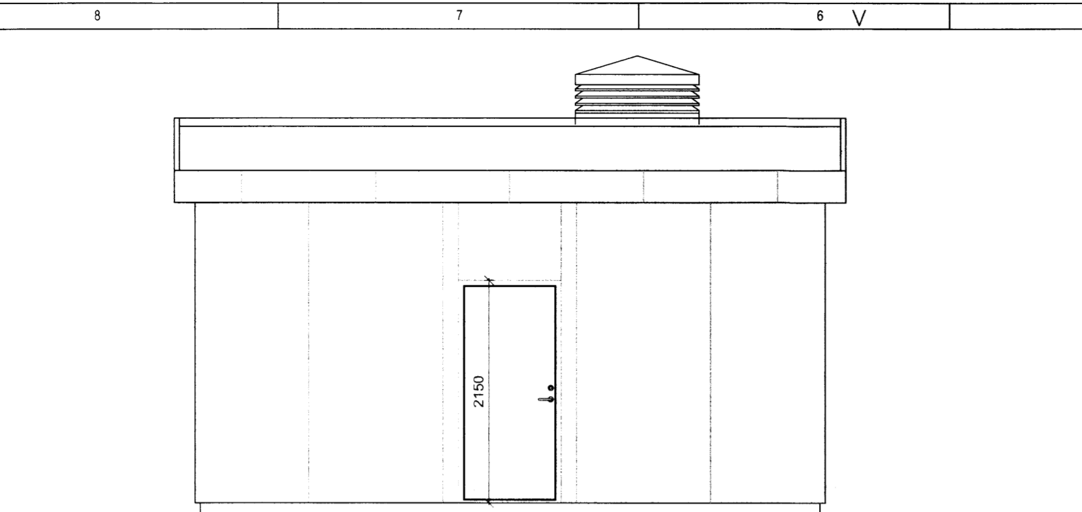
Suðurhlíð M 1:50
