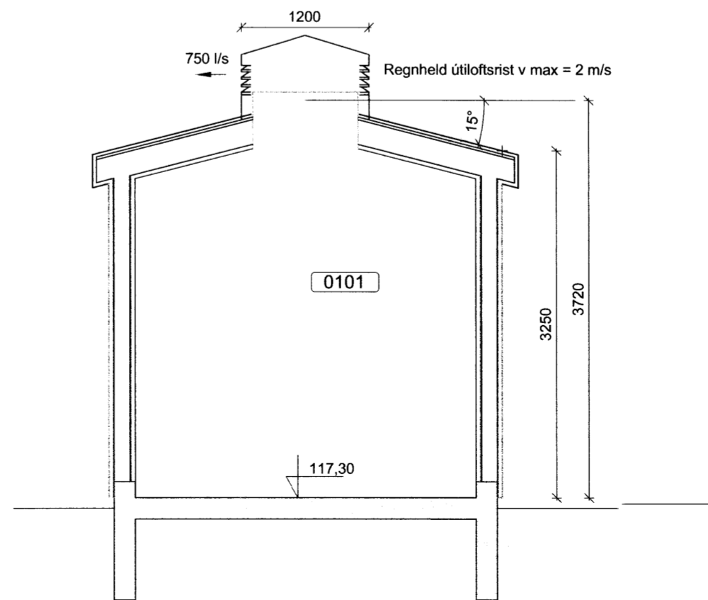
Sneiðing M 1:50
