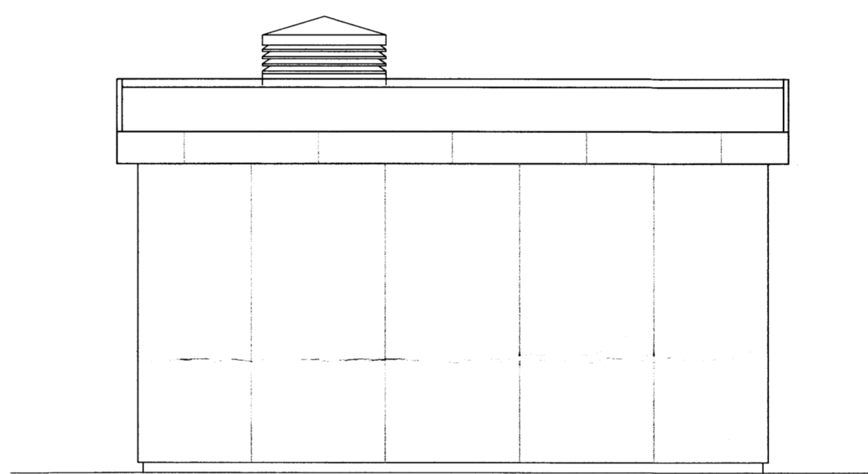
Norðurhlíð M 1:50
