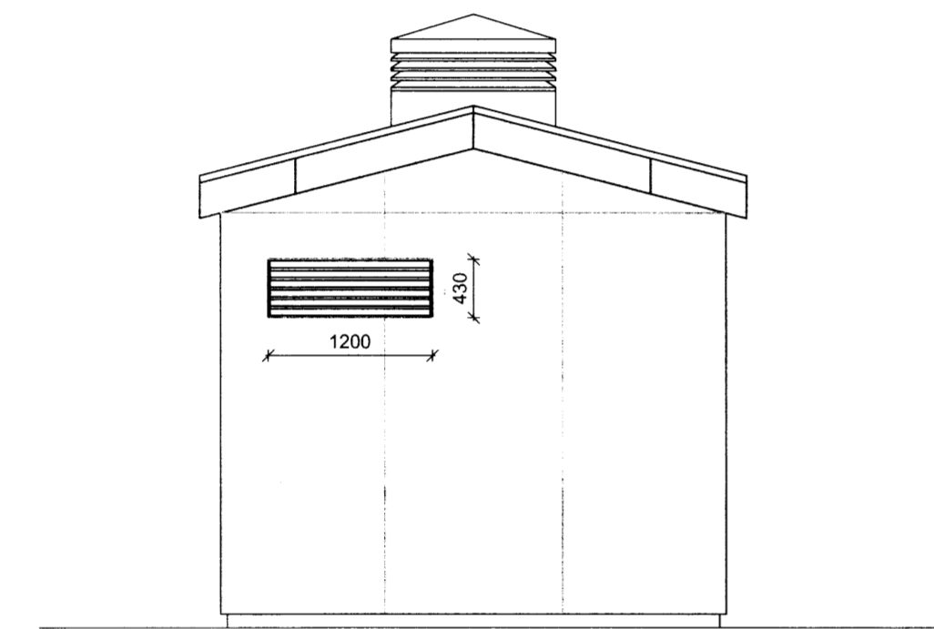
Vesturhlíð M 1:50
