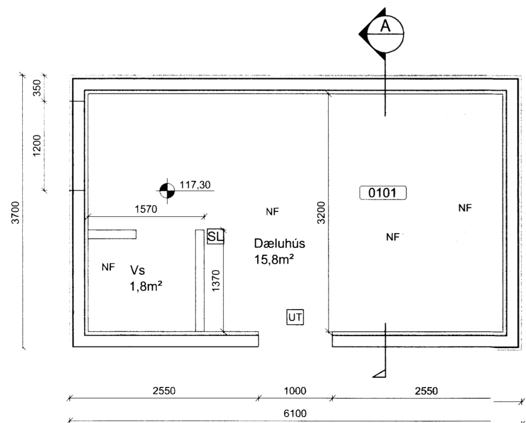
Grunnmynd M 1:50
