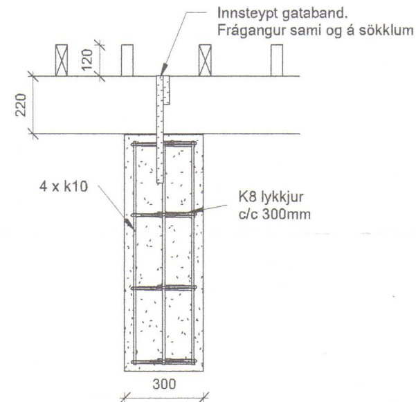
3 Snið í súlu undir pall 1 : 20
