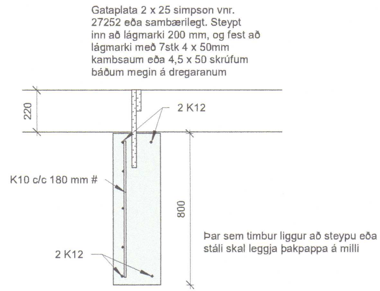
2 Snið í sökkul 1 : 20
