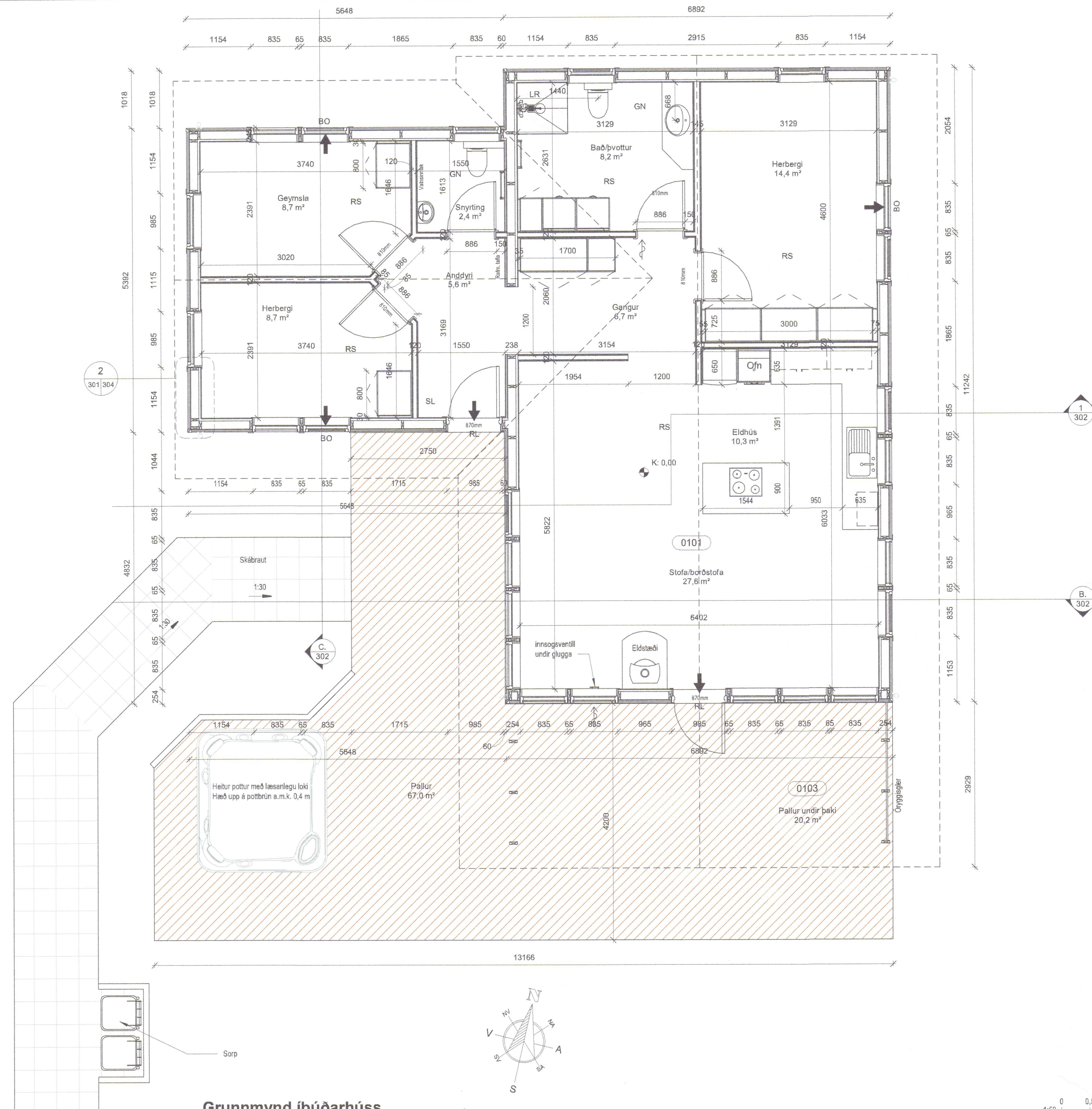
Grunnmynd íbúðarhúss. 1 : 50
