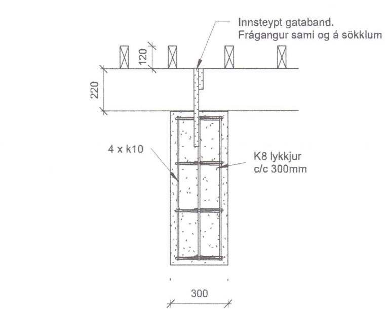
3 201/201 Snið í súlu undir pall 1 : 20
