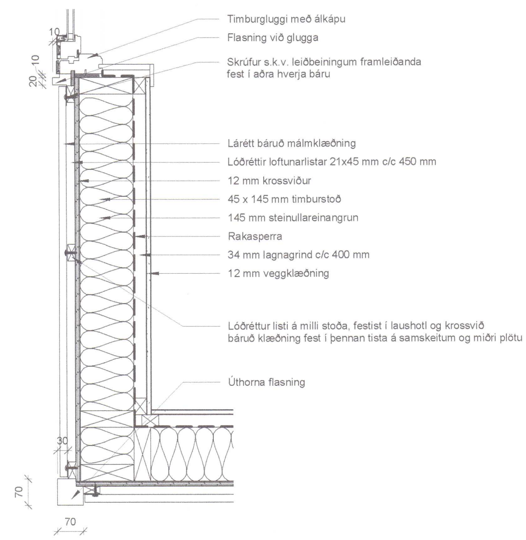
2 Deili C - Lárétt deili í útvegg 301 304 1 : 10
