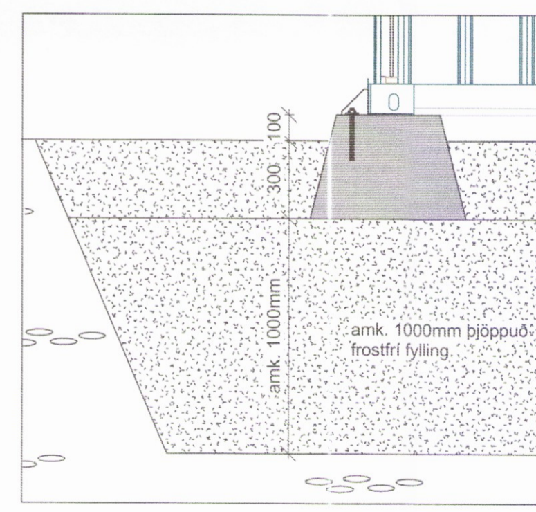
Snið A 1 : 20
