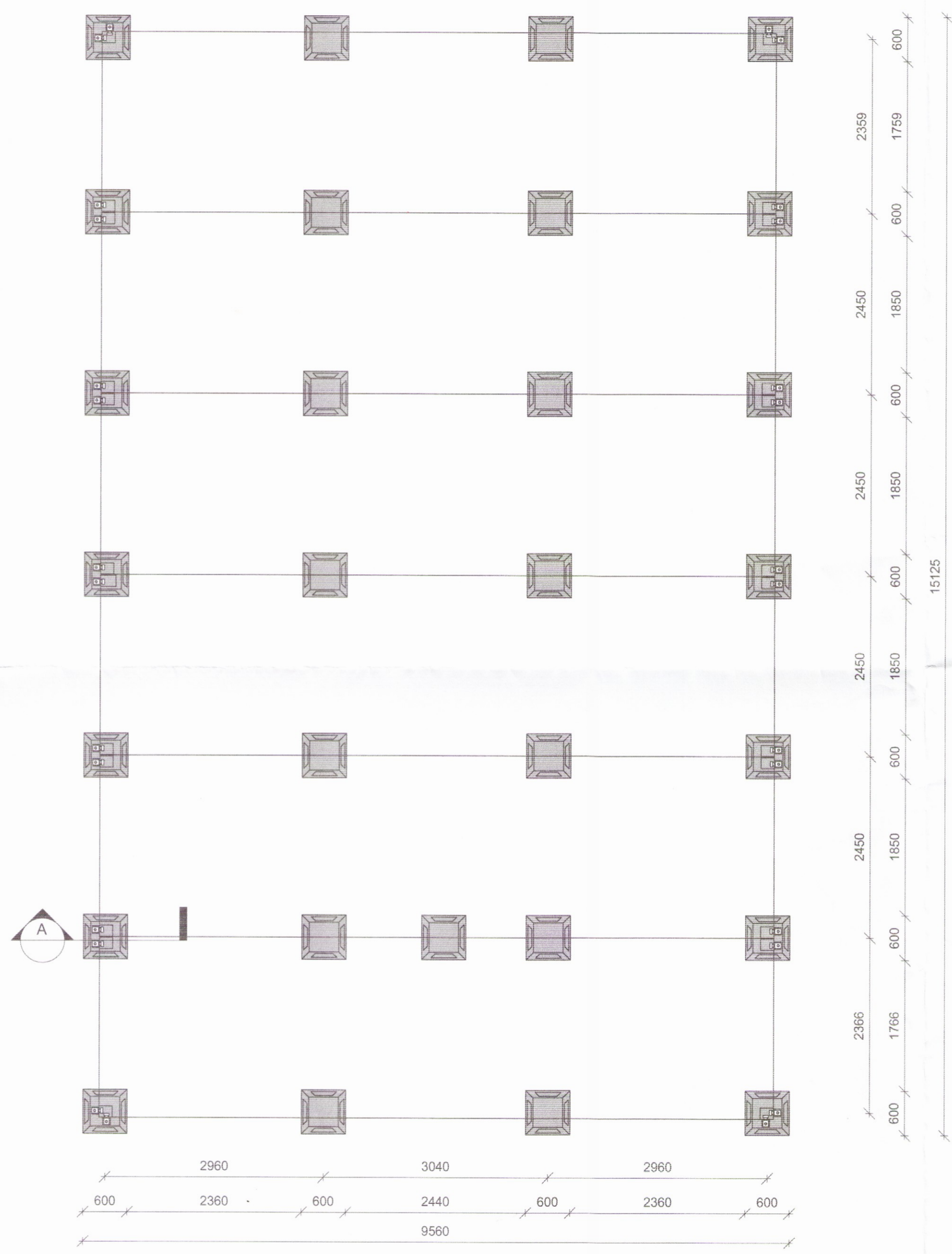
Grunnmynd undirstaða 1 : 50
