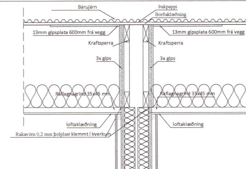
Lóðrétt sneið í útvegg mkv. 1:20
