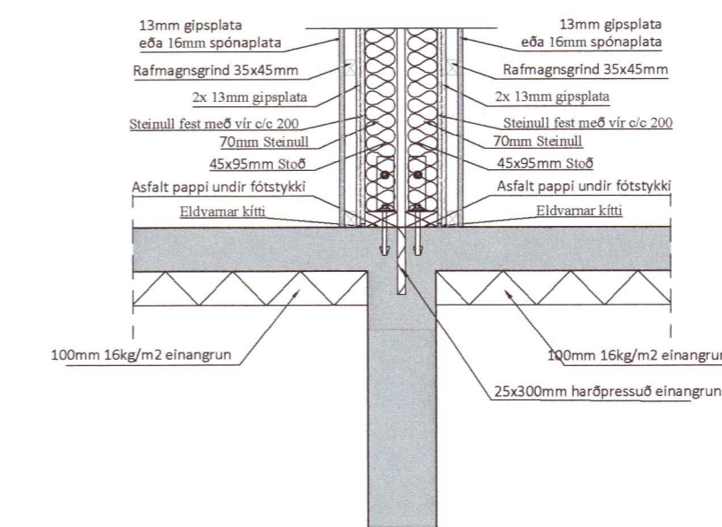
Lóðrétt sneiðing í millivegg (fótstykki) milli íbúða EI90 mkv.1:20
