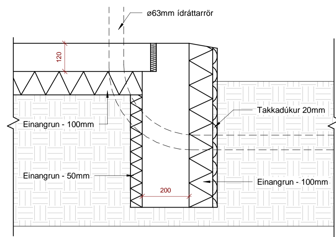
2 ÍDRÁTTARRÖR 1 : 10
