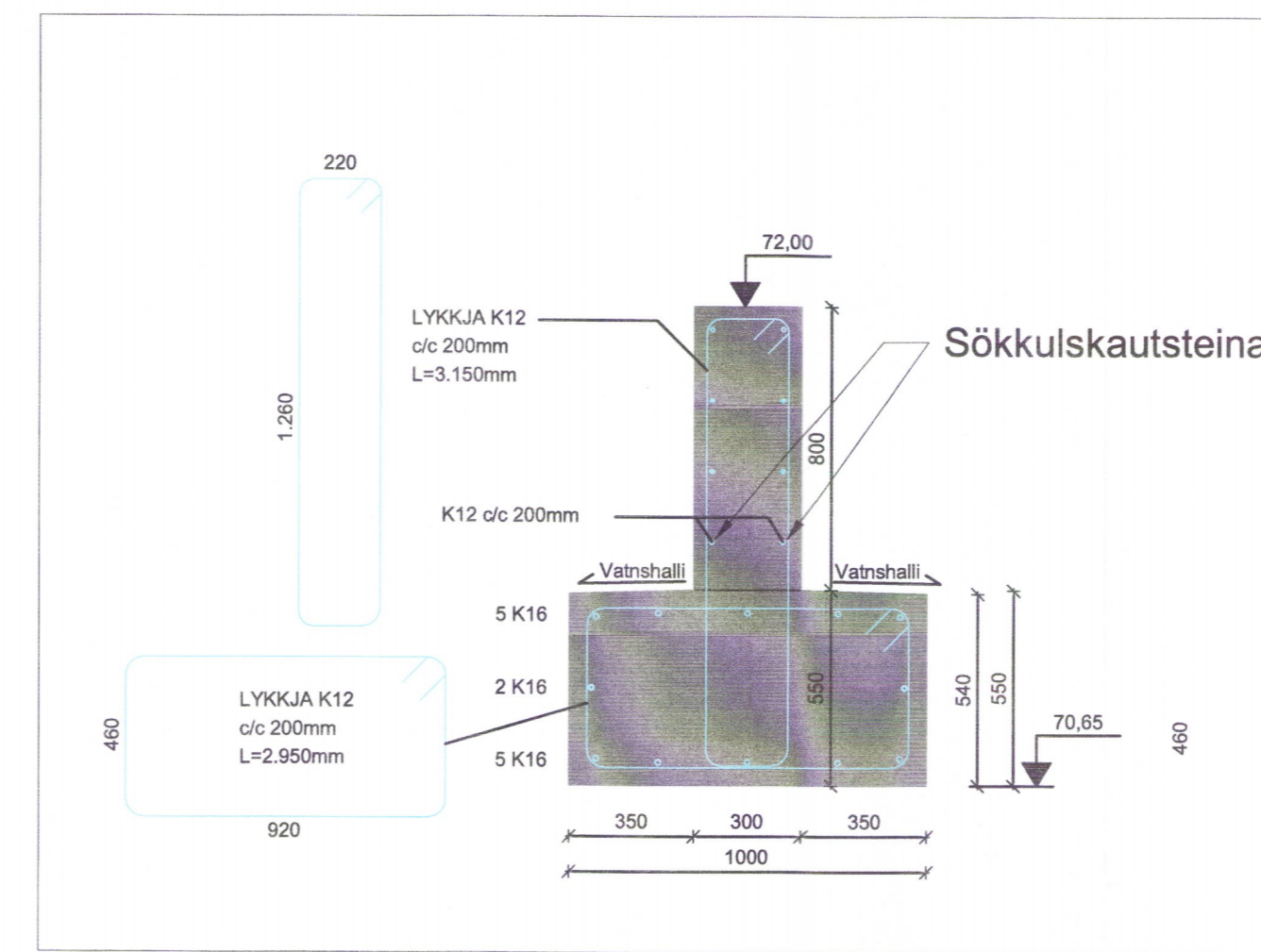
Snið af sökkli
