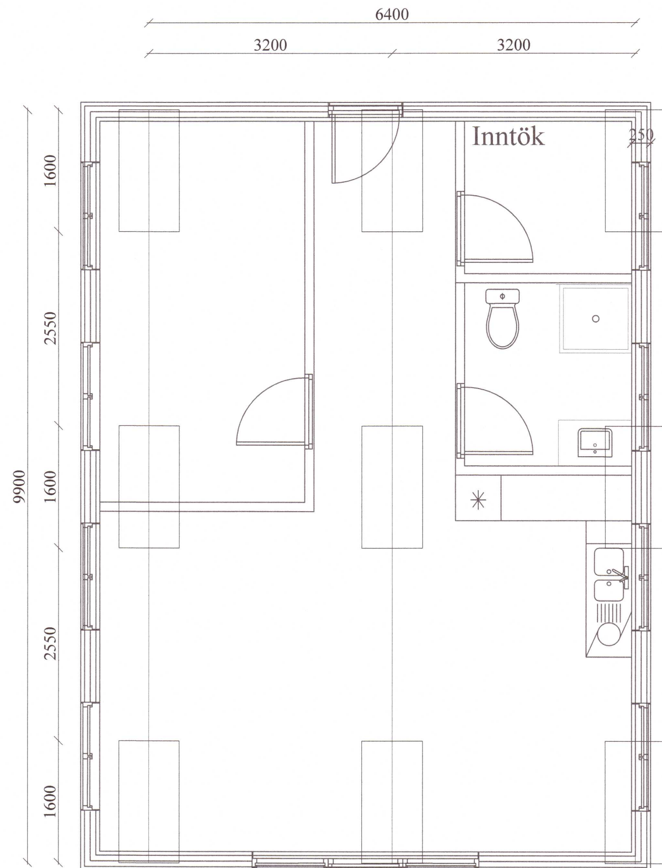
Grunnmynd undirstaðna 1:50
