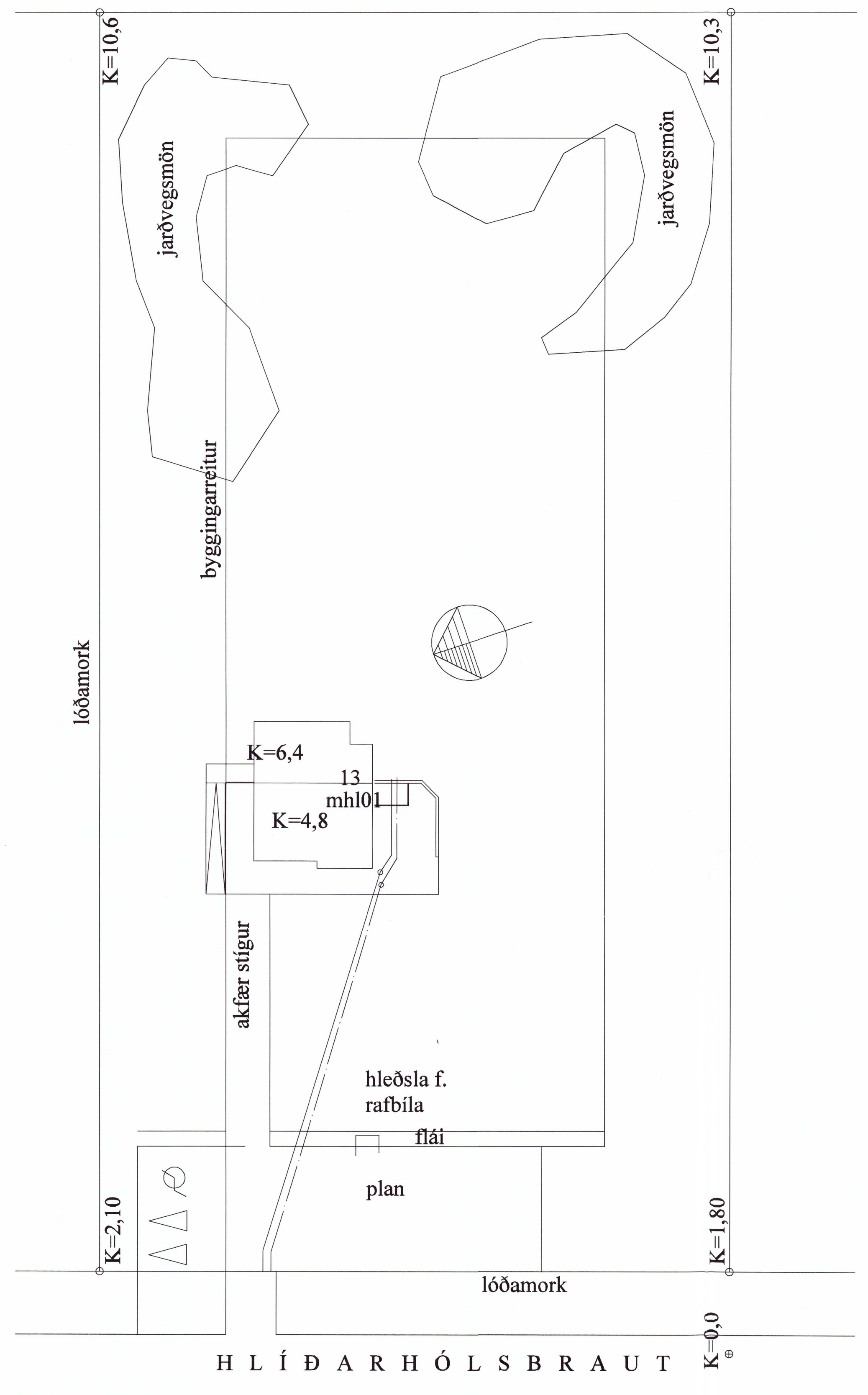
Afstöðumynd, 1:500
