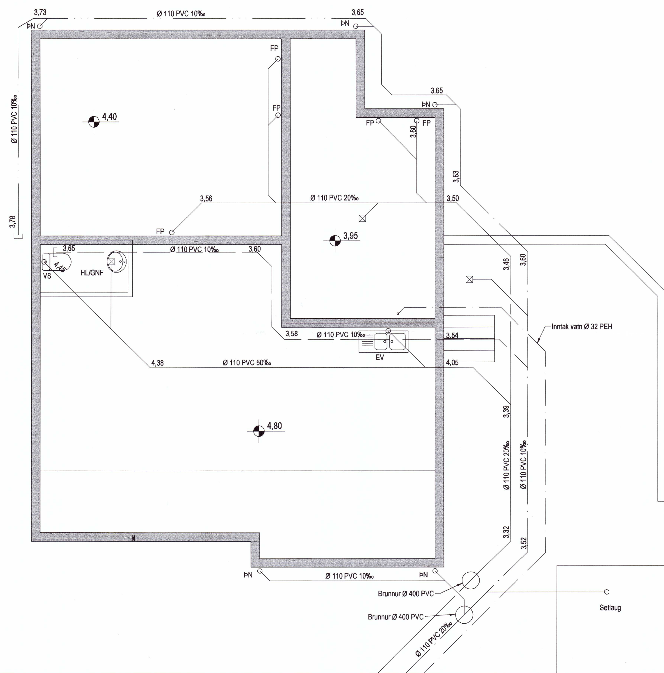
Fráveitulagnir, Grunnmynd, 1:50
