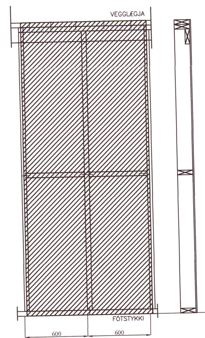
UPPBYGGING ÚTVEGGJA Mkv. 1:20
