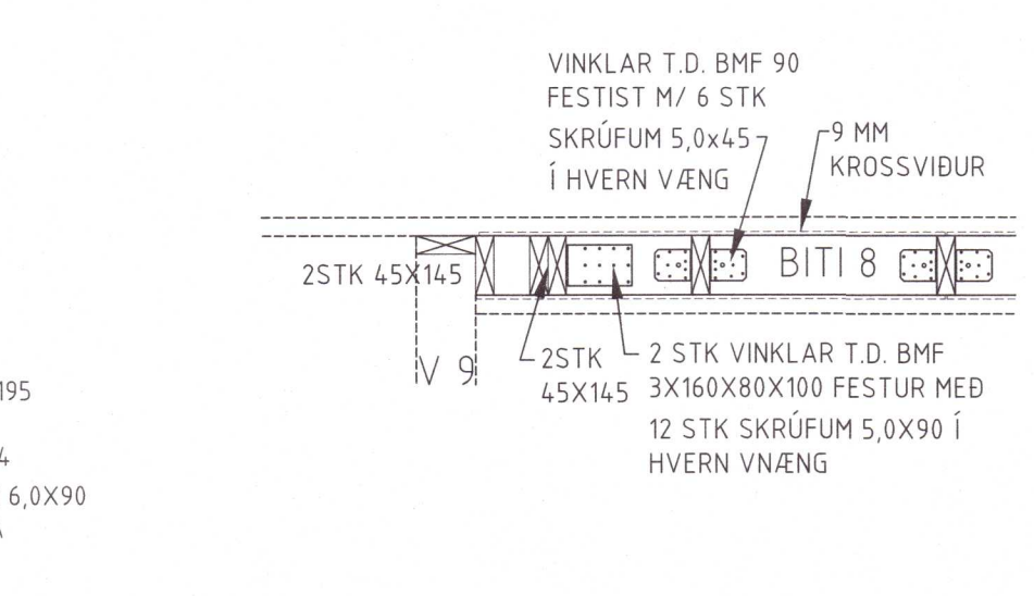
D65 DEILI 106 107 1:20
