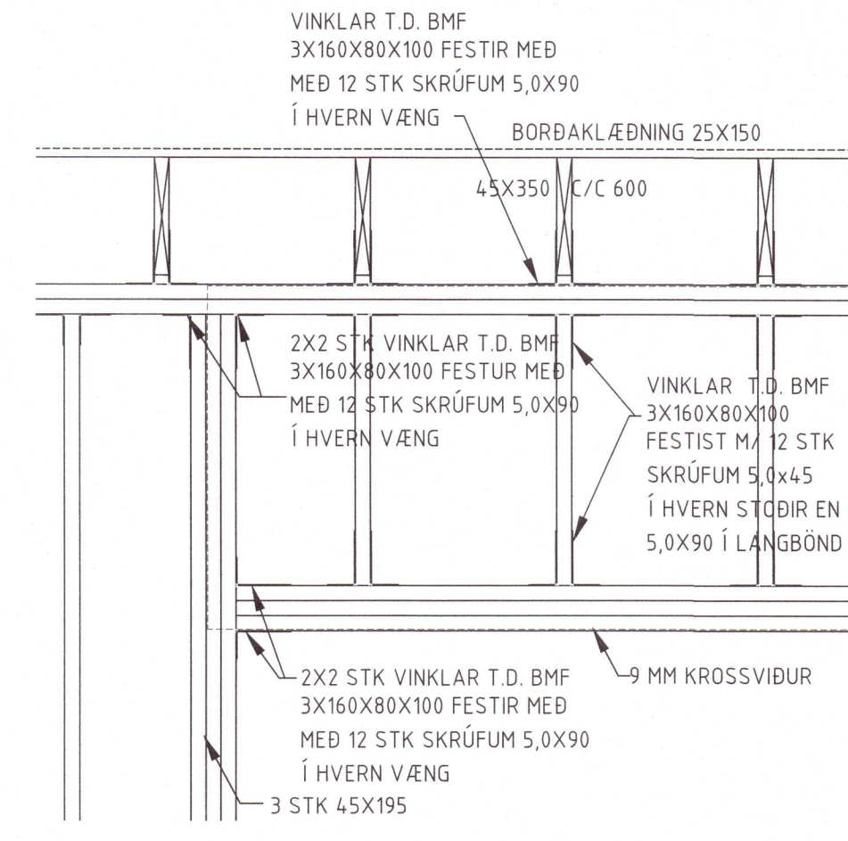
D52 DEILI 106 107 1:20
