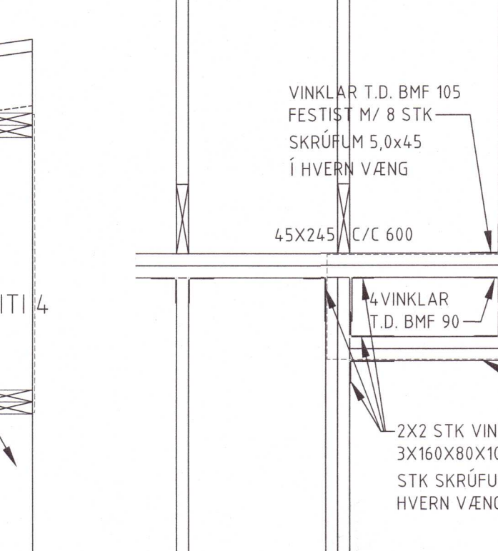
D68 DEILI 106 107 1:20
