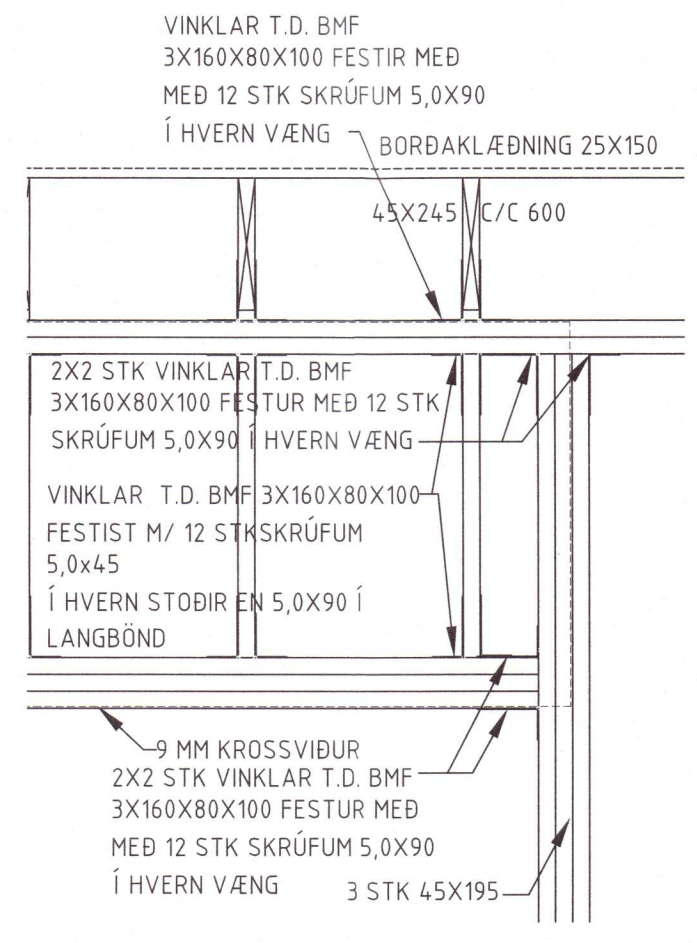
D54 DEILI 106 107 1:20
