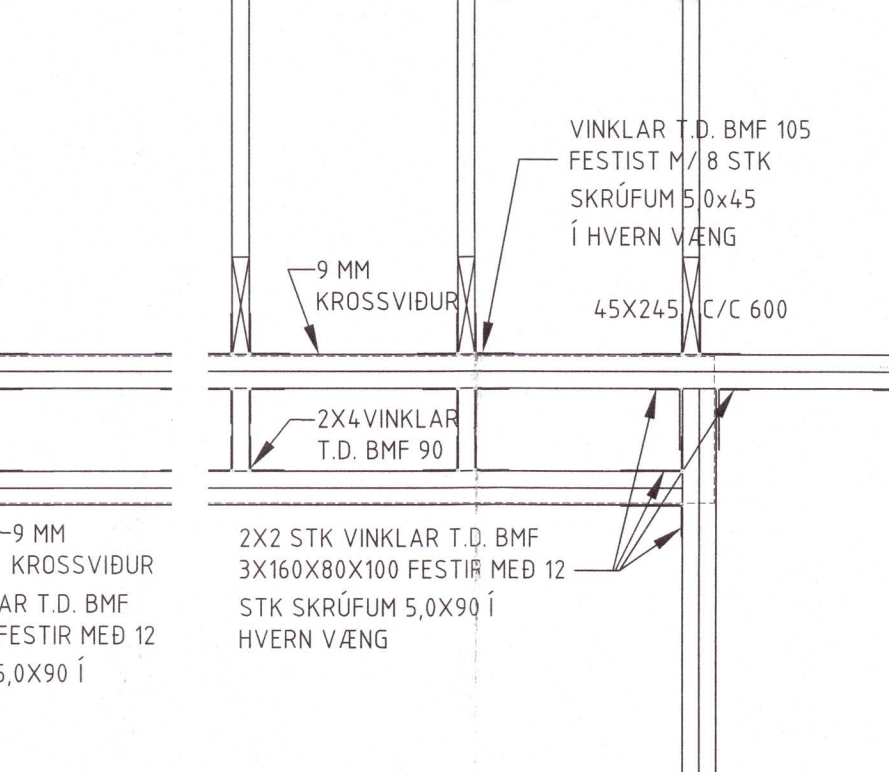
D70 DEILI 106 107 1:20
