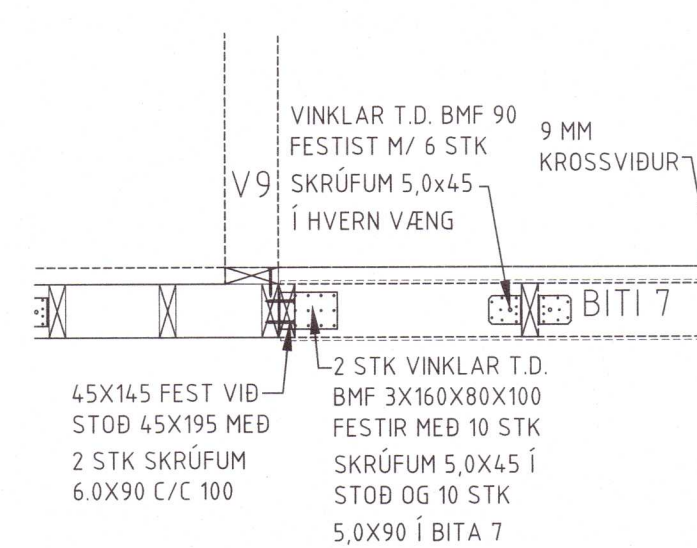
D61 DEILI 106 107 1:20
