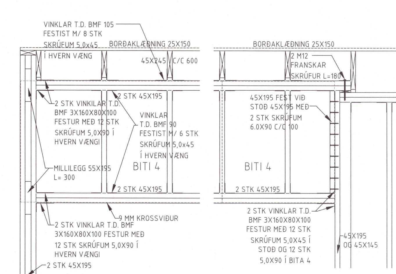
D48 DEILI 106 107 1:20
