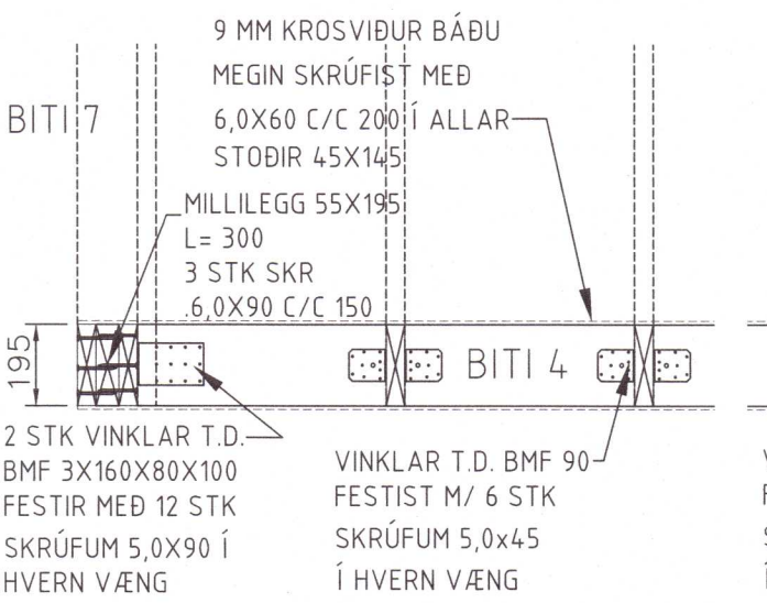
D49 DEILI 106 107 1:20
