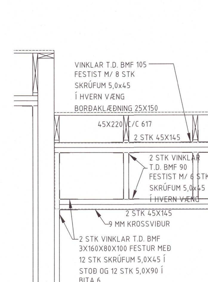
D56 DEILI 106 107 1:20
