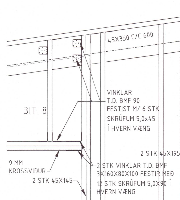
D66 DEILI 106 107 1:20
