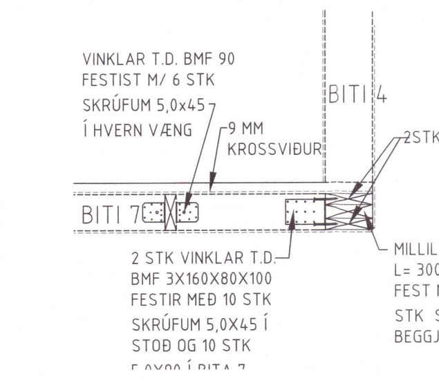
D63 DEILI 106 107 1:20
