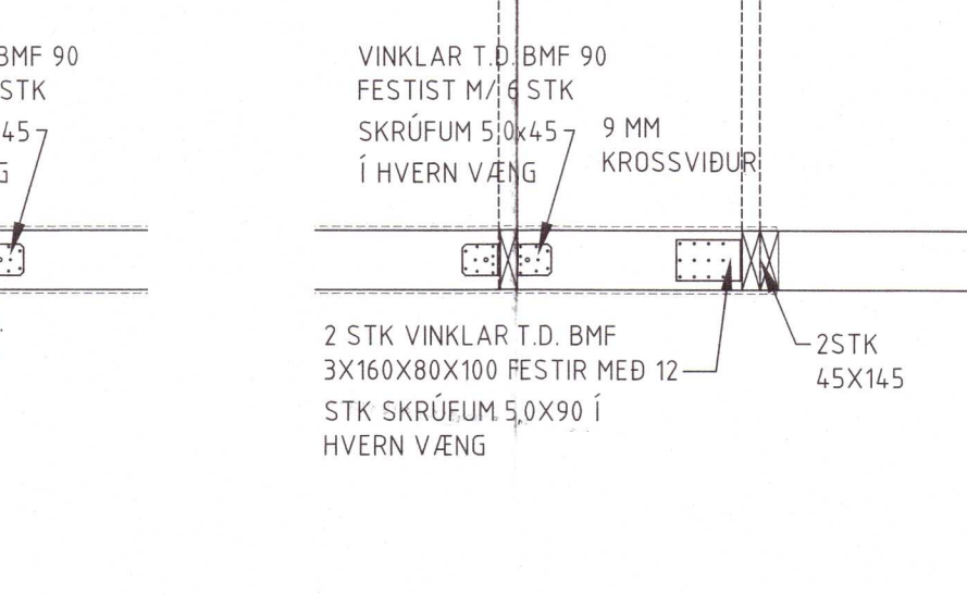
D71 DEILI 106 107 1:20
