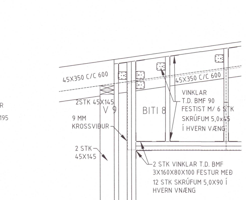
D64 DEILI 106 107 1:20
