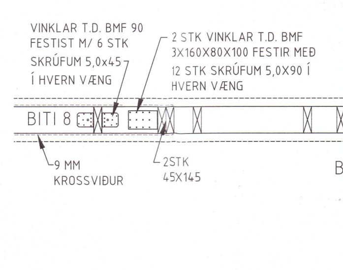
D67 DEILI 106 107 1:20
