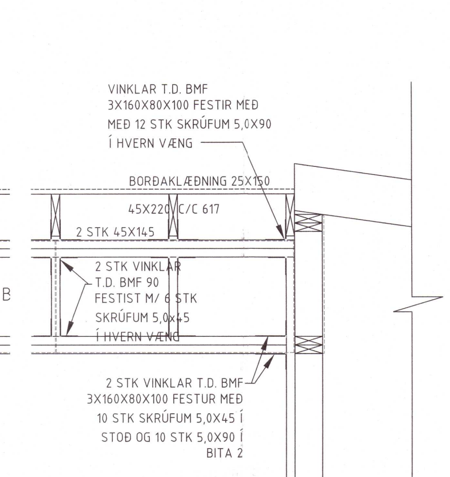
D58 DEILI 106 107 1:20
