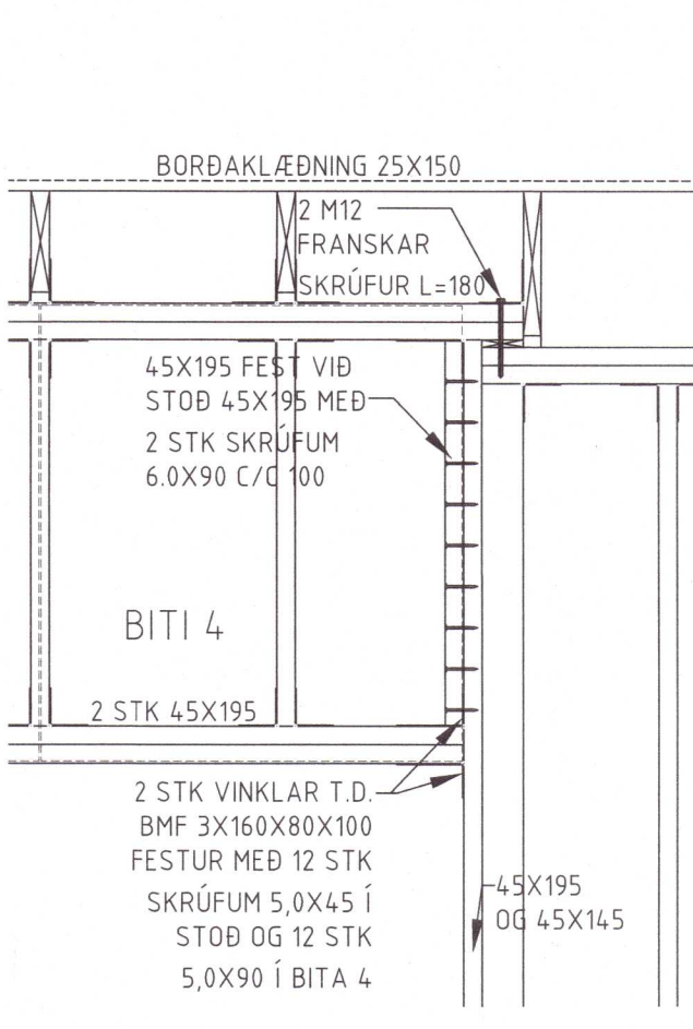
D50 DEILI 106 107 1:20
