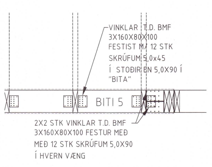
D55 DEILI 106 107 1:20
