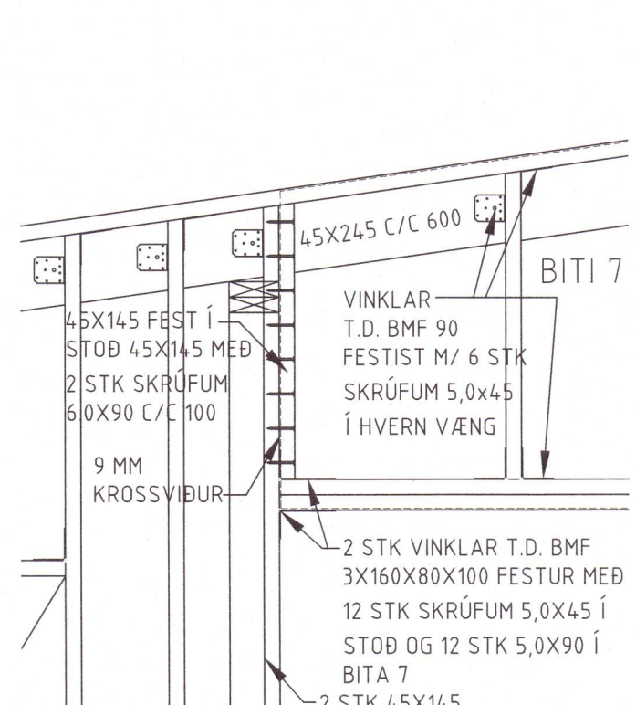
D60 DEILI 106 107 1:20
