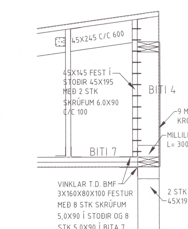
D62 DEILI 106 107 1:20
