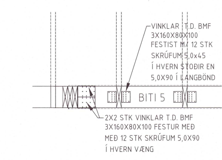
D53 DEILI 106 107 1:20
