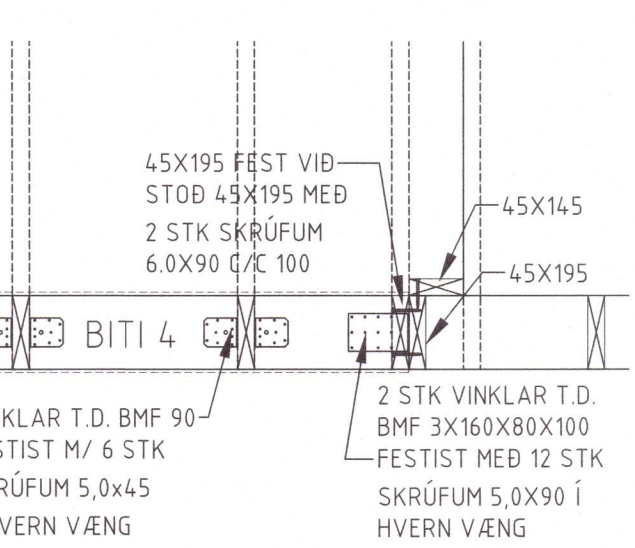
D51 DEILI 106 107 1:20
