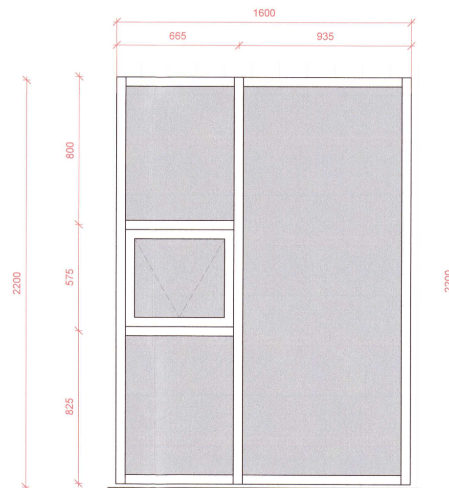
5 G5 1:20 1 stk
