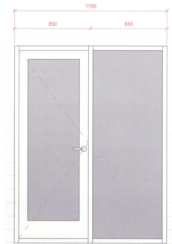
4 G4 1:20 1 stk
