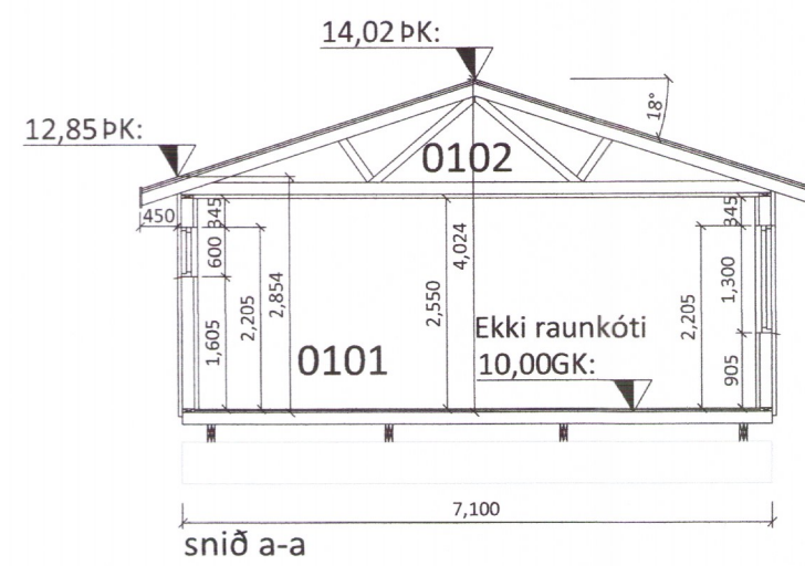
snið a-a
