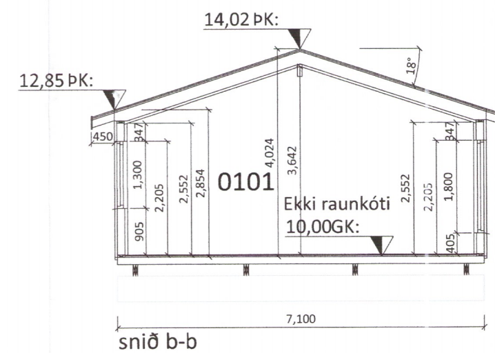
snið b-b
