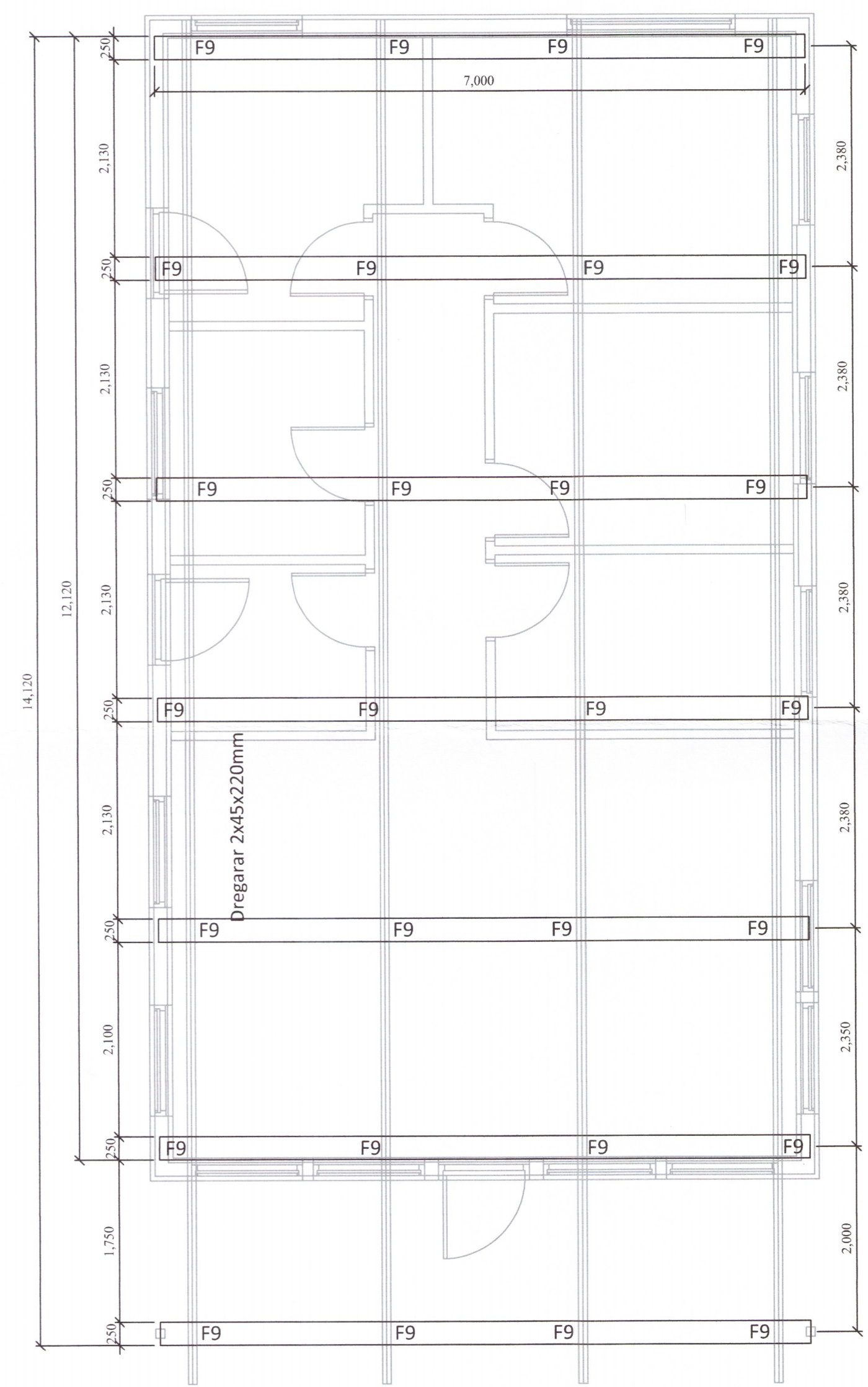
Grunnmynd steyptra þverveggja og festinga mkv. 1:50
