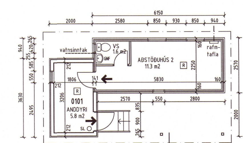
ABSTÖÐUHÚS 2 MHL 02 1:100
