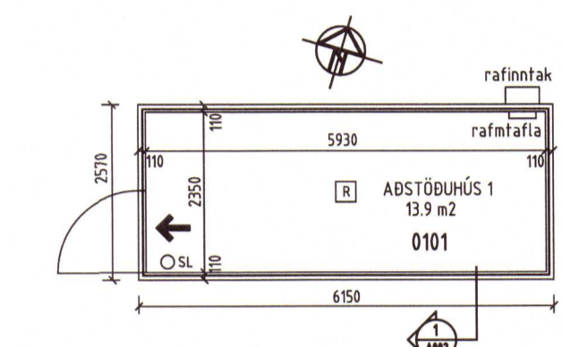
ABSTÖÐUHÚS 1 MHL 01 1:100
