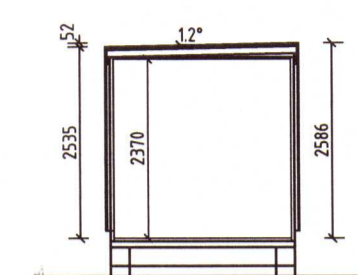
SNID 1-1 1:100
