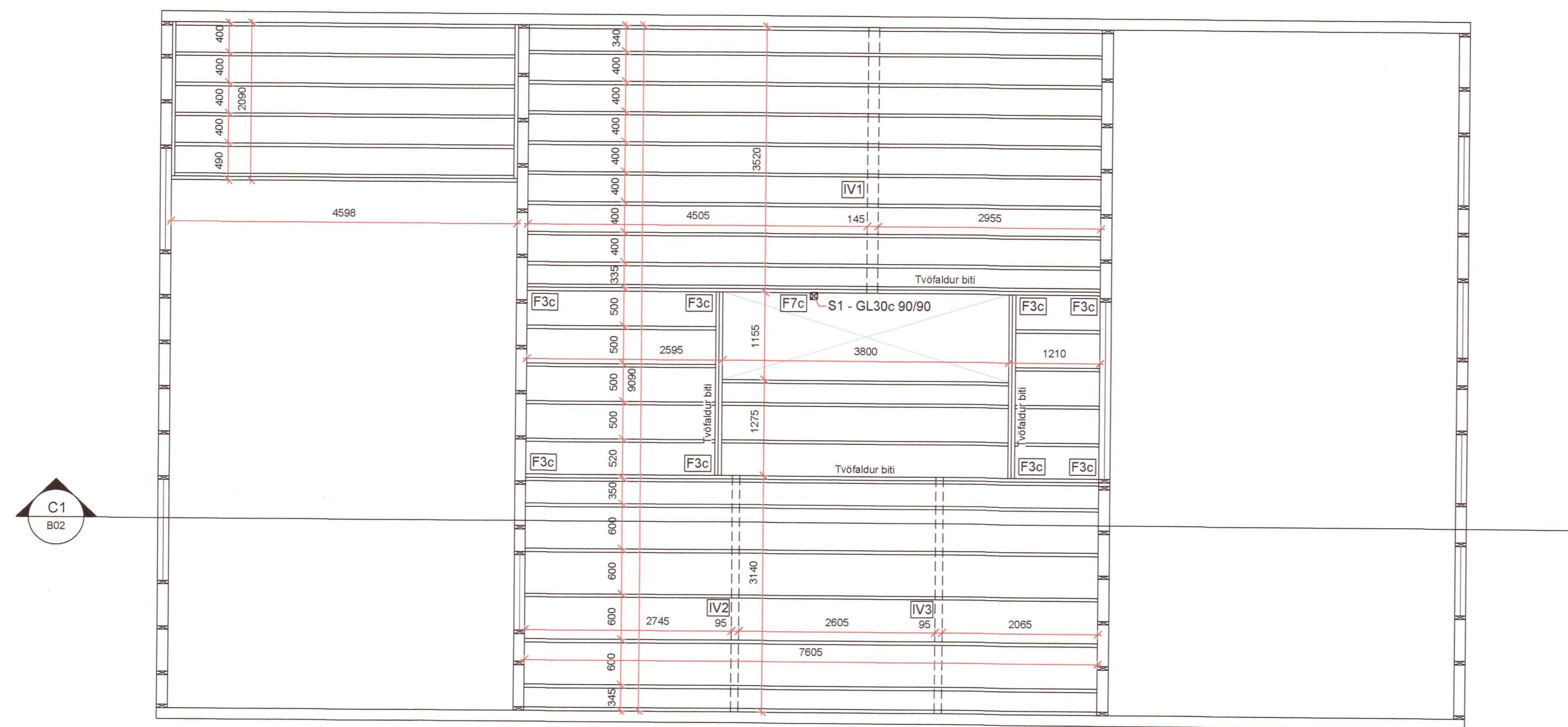
GRUNNMYND Mkv. 1:50
