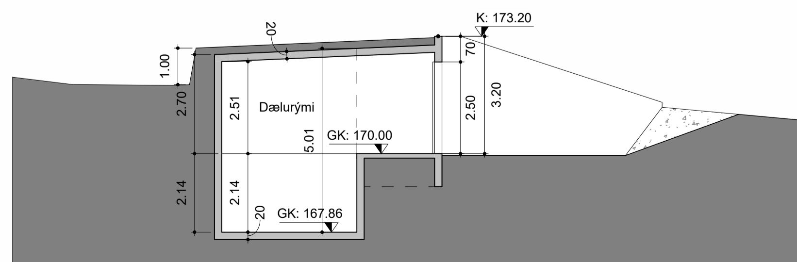
Snið B 1:100
