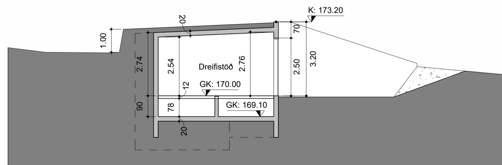
Snið A 1:100
