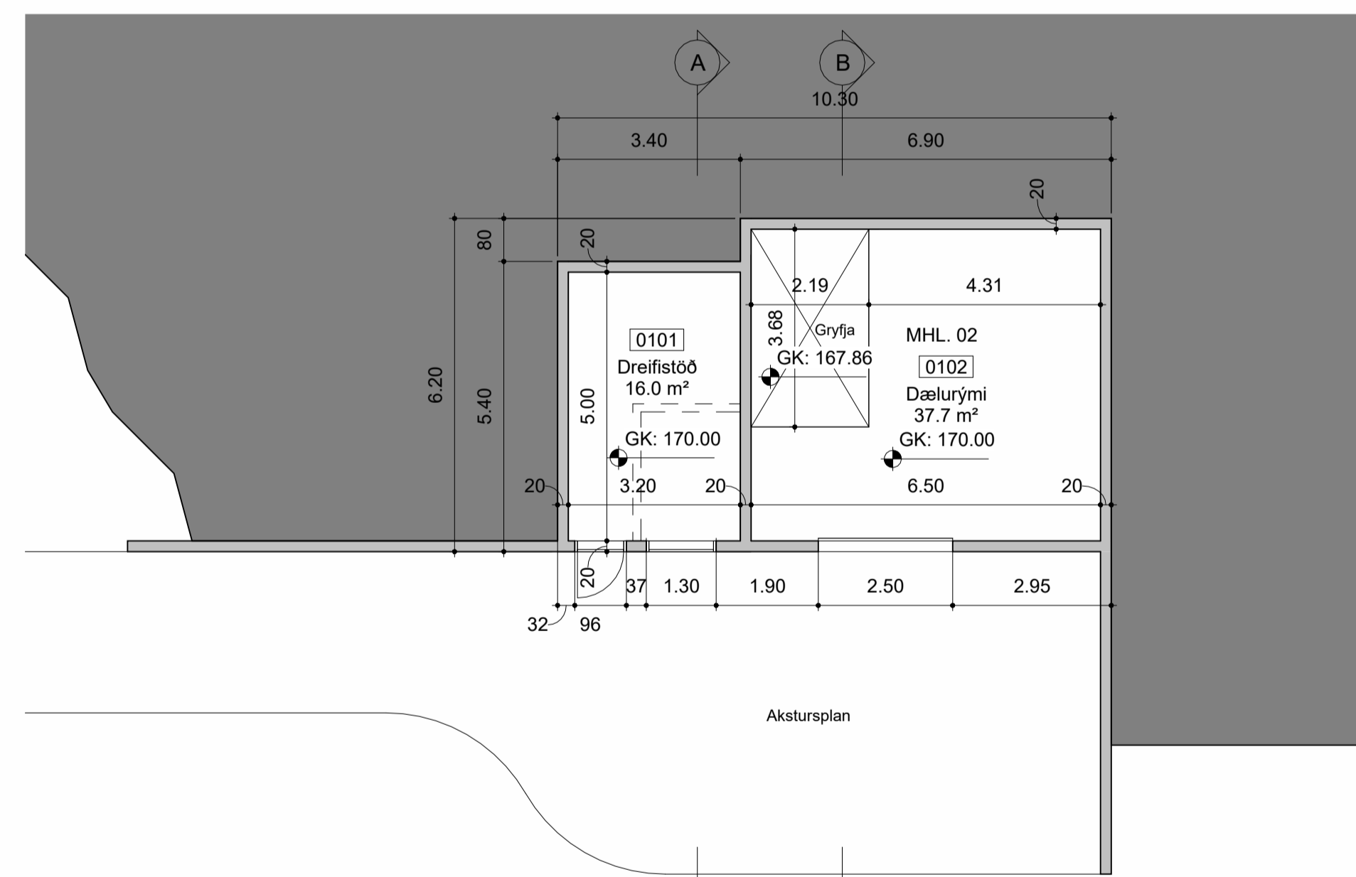
Grunnmynd 1. Hæðar 1:100
