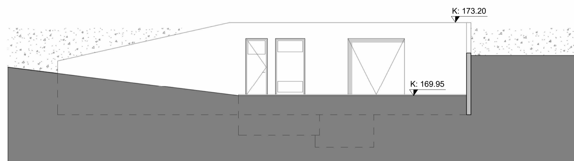
Ásýnd í suður 1:100
