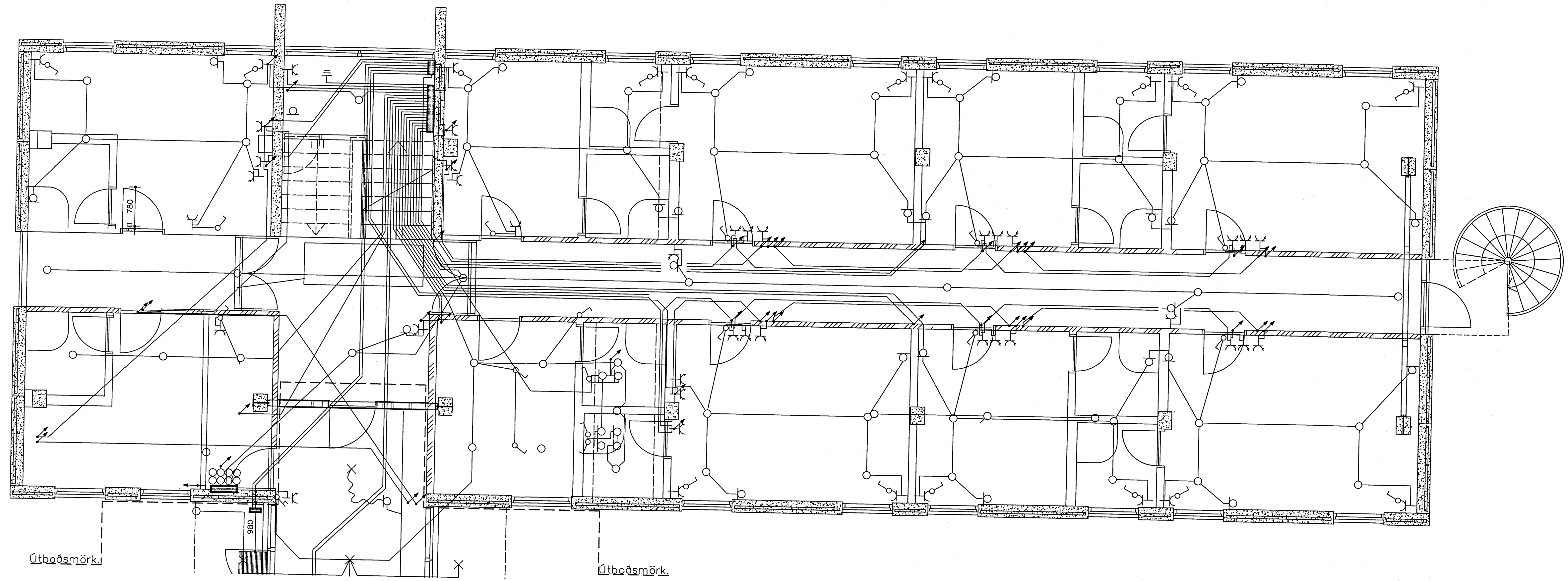
GRUNNMYND 1.HÆÐ
