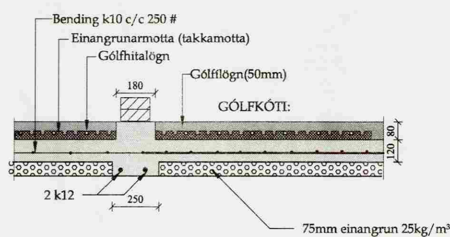
03 Snið 03 1-01 1-01 Mk. 1:20
