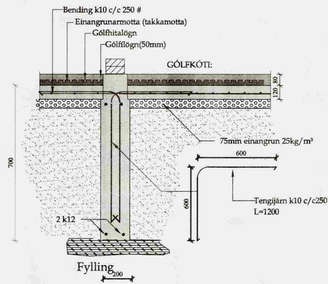
02 Snið 02 1-01 1-01 Mk. 1:20
