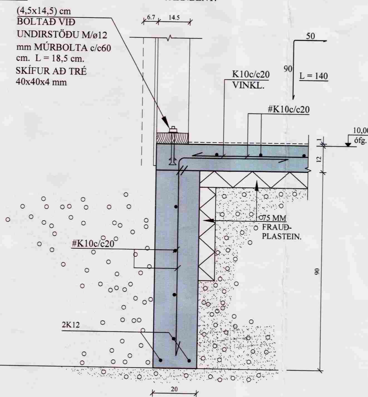
A2 SNID. 1:10 1-02 SNID A2' ER EINS JÄRNBENT.
