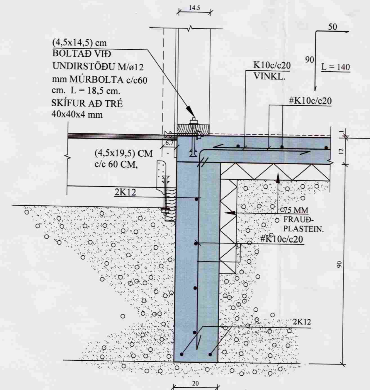
B2 SNID. 1:10 1-02 Í SNID B2' ER TENGT VIÐ NÚV. HÚS
