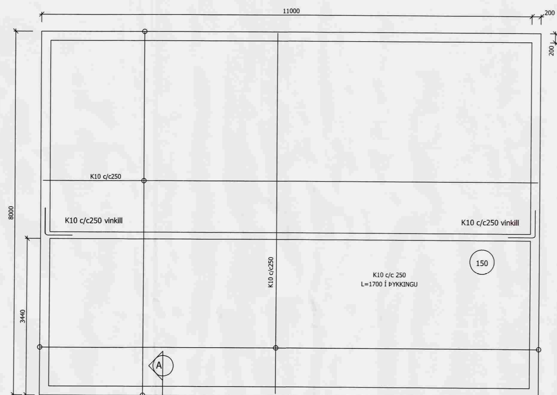
GRUNNMYND UNDIRSTADA Mkv 1:50
