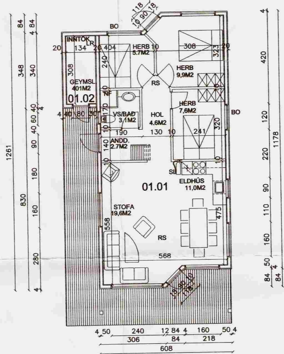
GRUNNMYND
