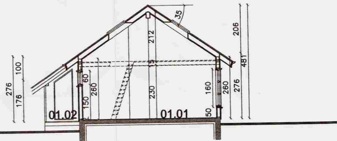
SKURÐUR A.
