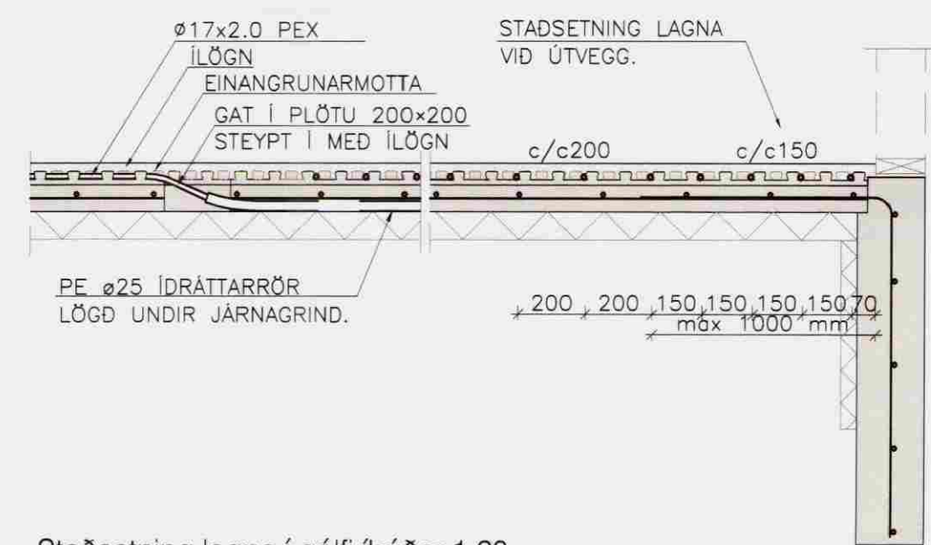
Staðsetning lagna í gólf í búðar 1:20
