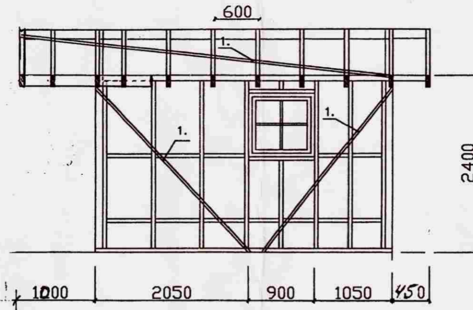
Vesturhlið 1:50
