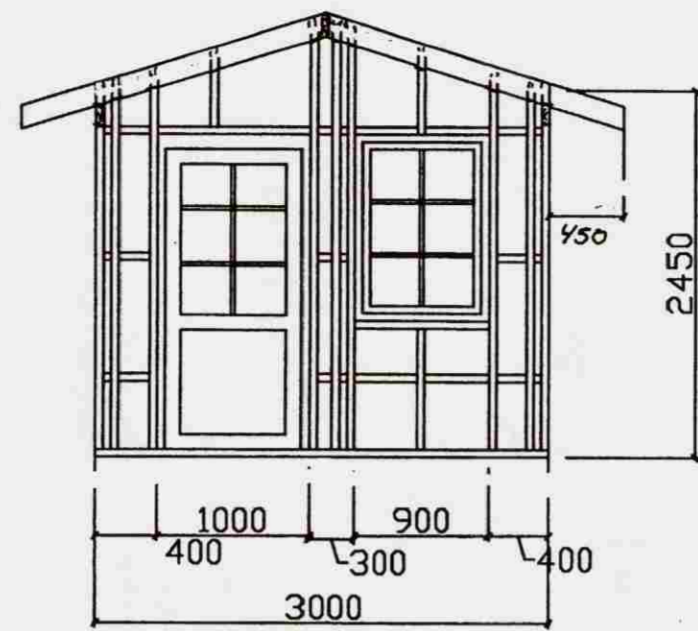
Suðurgafi 1:50
