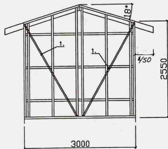
Norðurgafi 1:50
