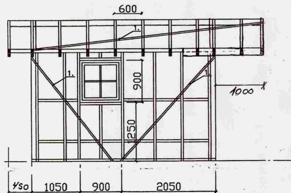
Austurhlið 1:50
