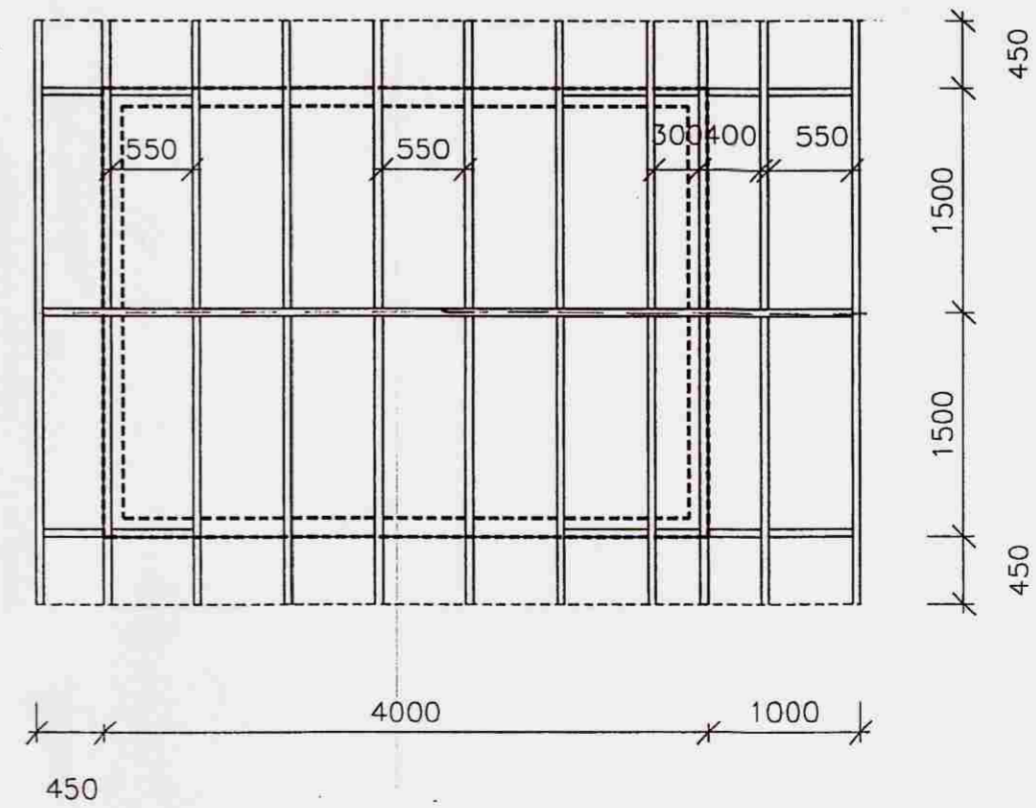
Pakviðir 1:50
