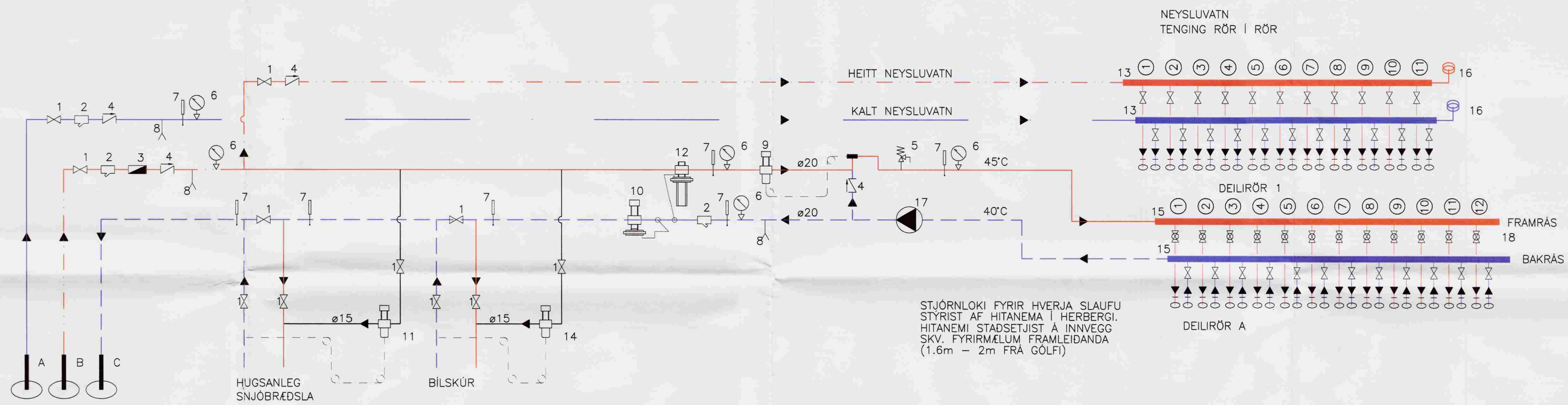
KERFISMYND HITÁ- OG NEYSLUVATNSKERFIS
