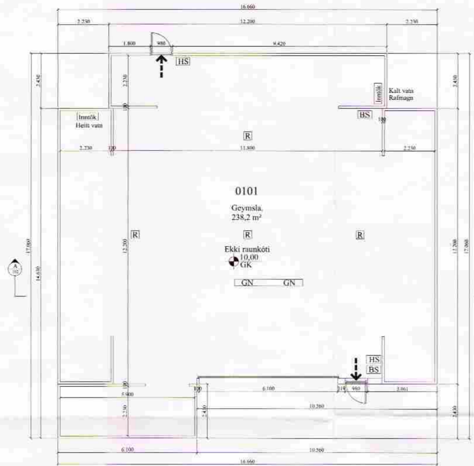
GRUNNMYND
