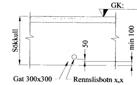
Skýringamynd af sökkulgötum
