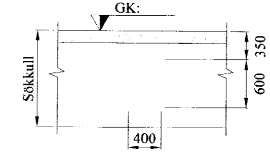
Skýringamynd af inntaksgati
