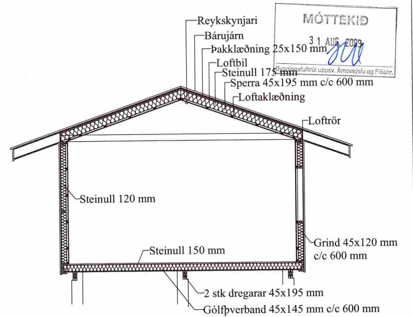
Snið A - A
