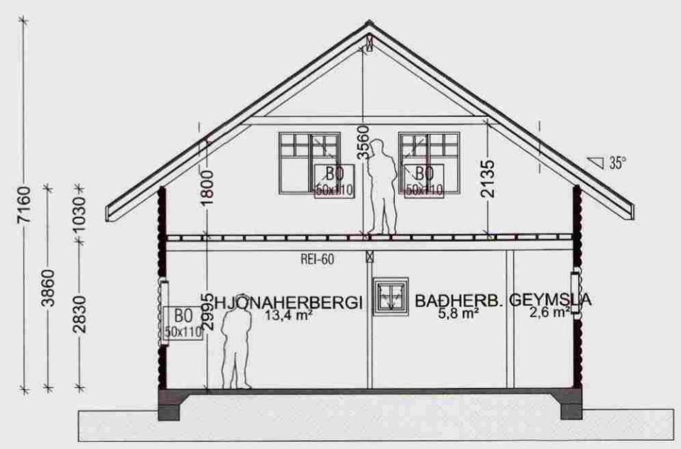
SNID A-A 1:100
