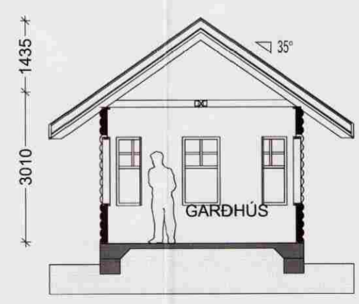
SNID B-B 1:100
