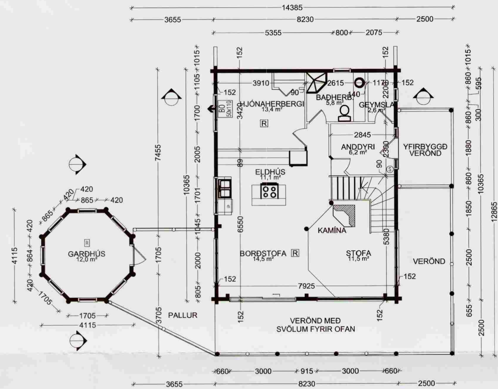
1. HÆÐ GRUNNMYND 1:100
