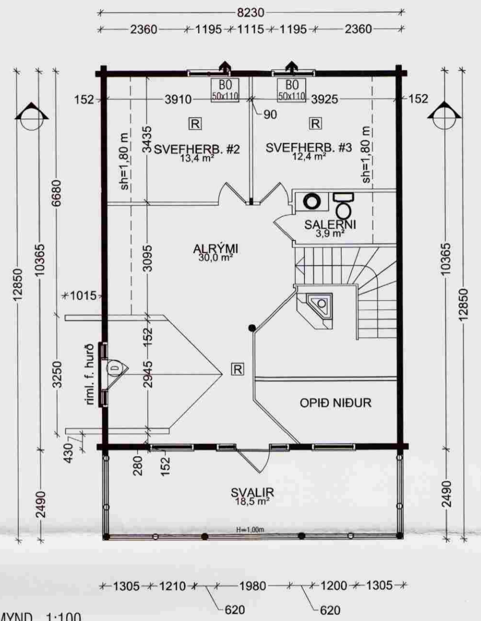
2. HÆÐ GRUNNMYND 1:100
