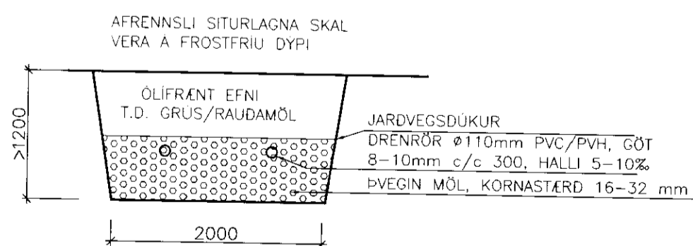
SITURLÖGN, SNIÐ Mkv. 1:50
