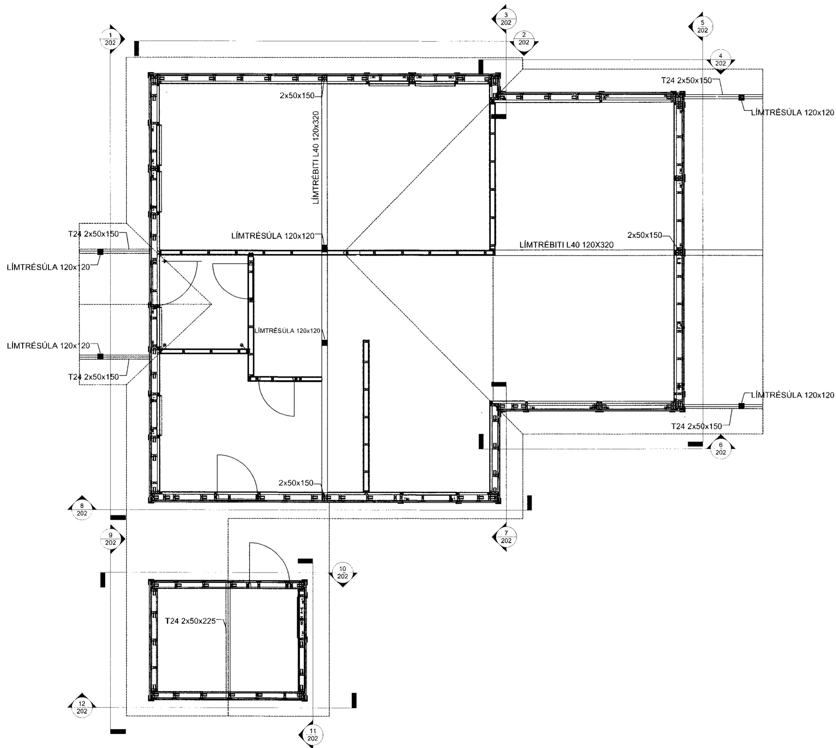
1 Grunnmynd 1 : 50
