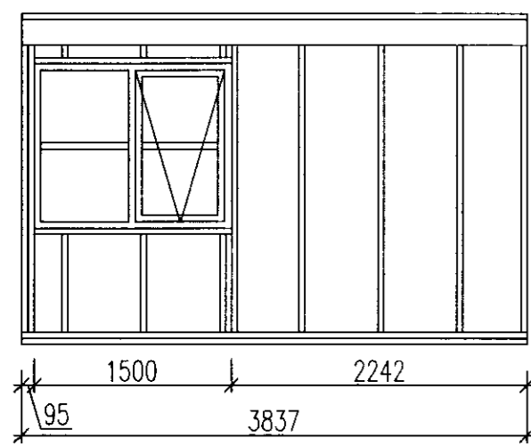
4 Snið 1 : 50
