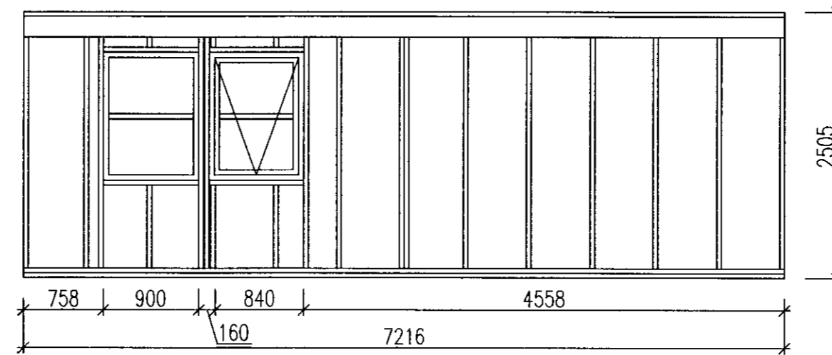
2 Snið 1 : 50
