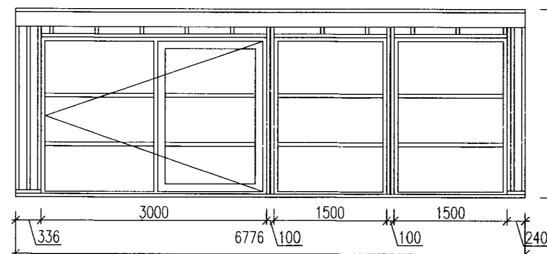
5 Snið 1 : 50
