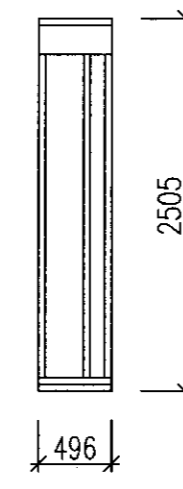
3 Snið 1 : 50
