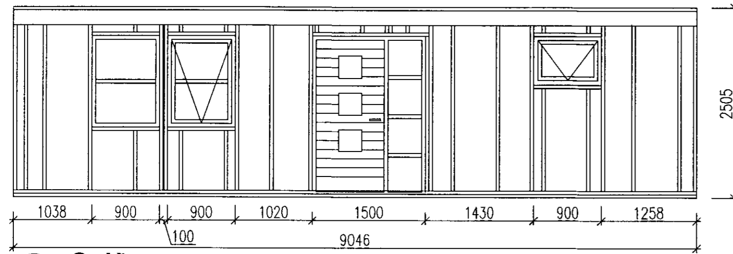
1 Snið 1 : 50
