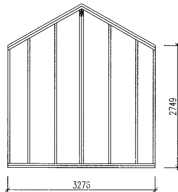
12 Snið 1 : 50
