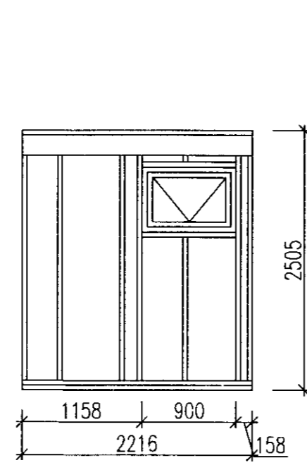
11 Snið 1 : 50
