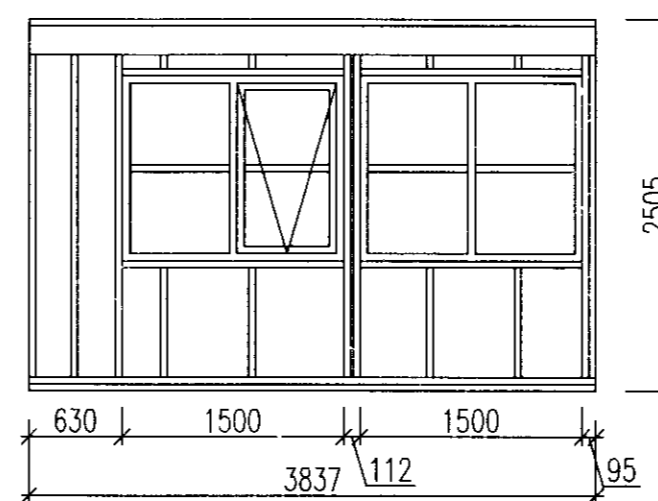
6 Snið 1 : 50
