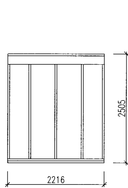
9 Snið 1 : 50
