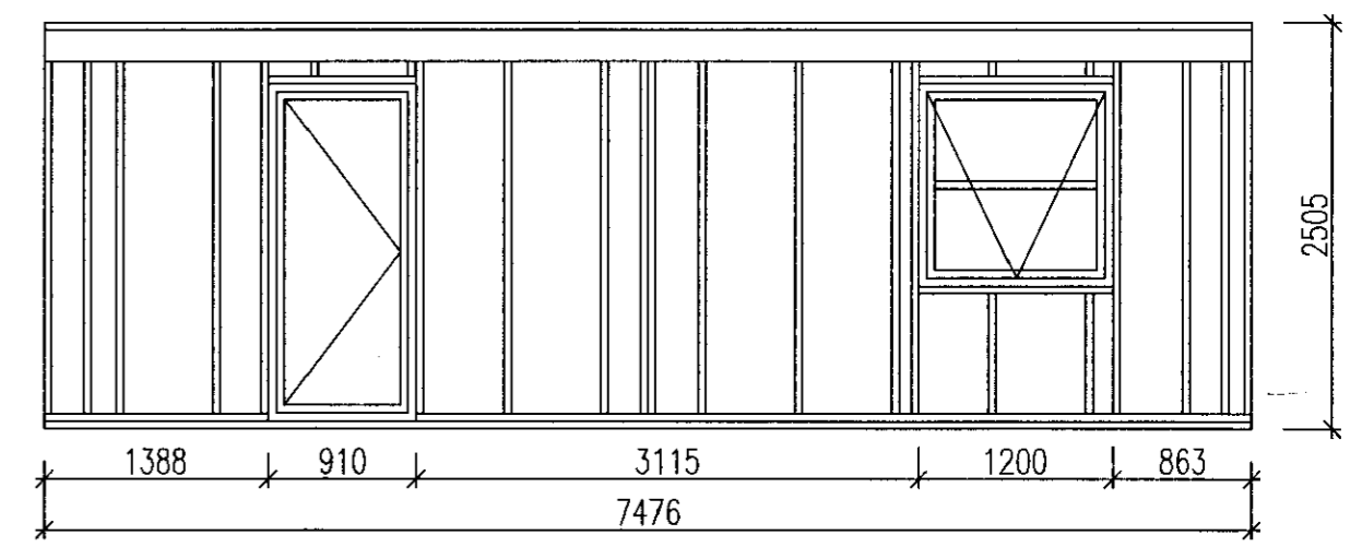
8 Snið 1 : 50
