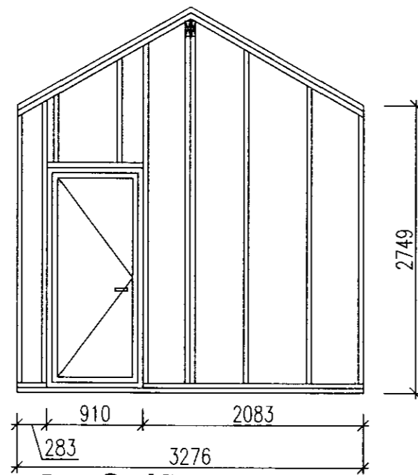
10 Snið 1 : 50
