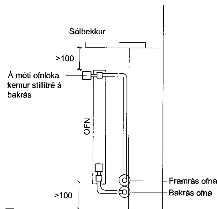
Ofnalagnir í vegg M 1:20
