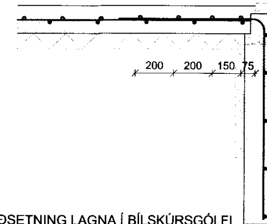
STAÐSETNING LAGNA Í BÍLSKÚRSGÓLFI 1:20
