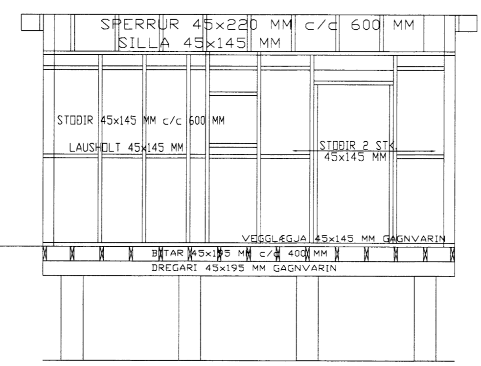
SNID - B 1:50
