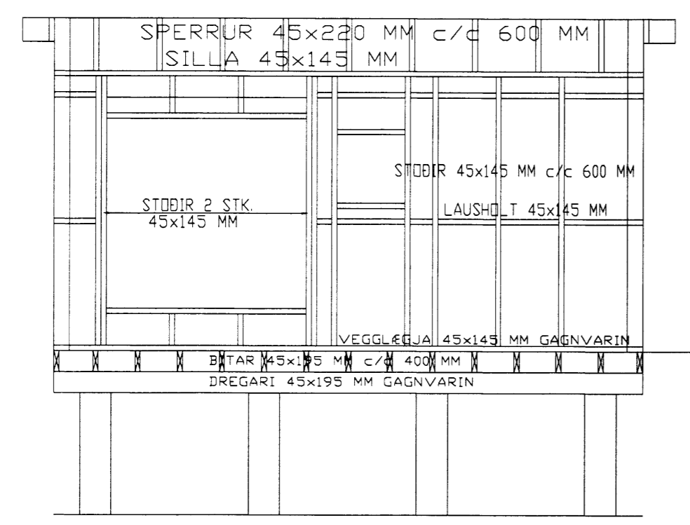
SNID - A 1:50
