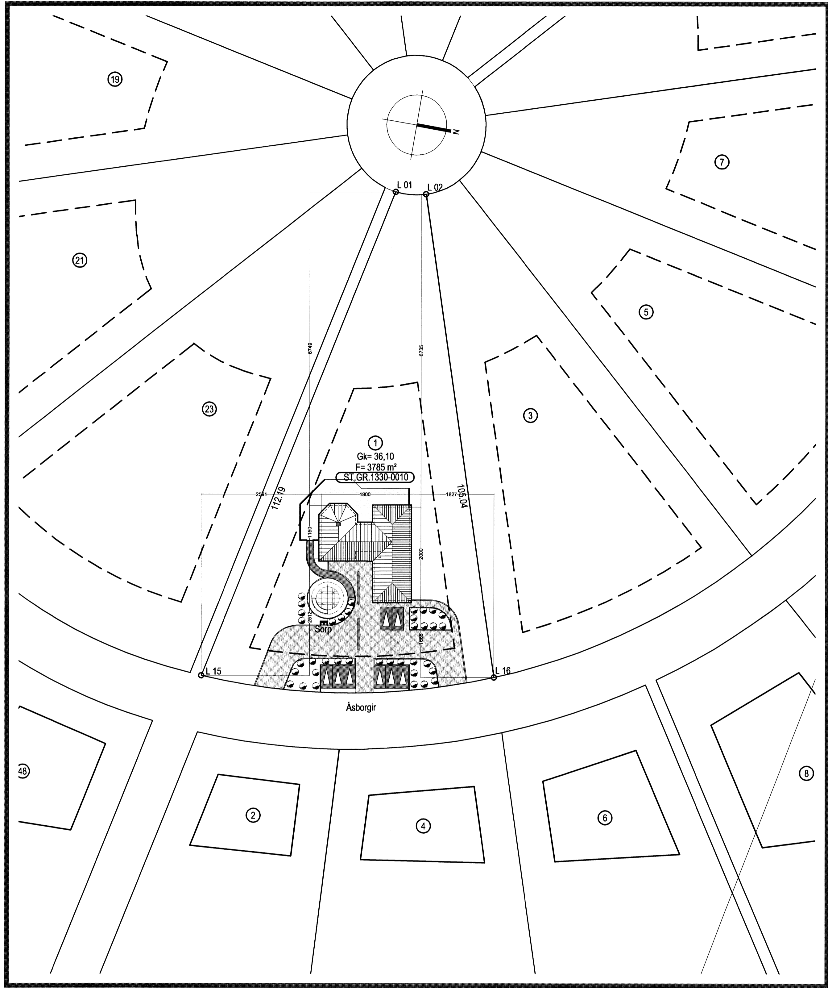
Afstöðumynd 1:500
