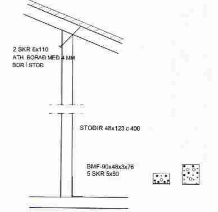
FESTING STÖDA VIÐ GÓLF- OG YFIRBAND
