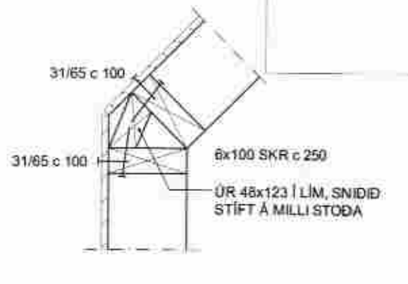
SAMSETNING Á 135° ÚTHORNI
