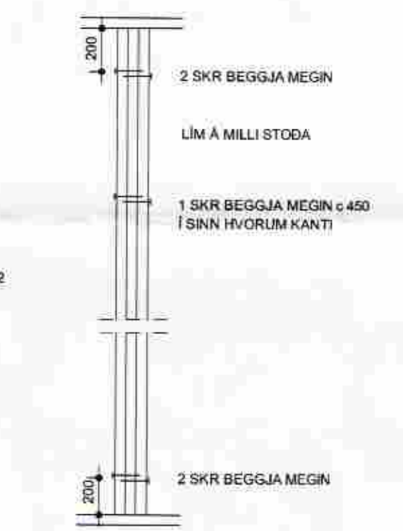
SAMSETNING Á 2- OG 3-FÖLDUM STÖÐUM, 4-FALDAR STÖÐIR BOLTA SAMAN, SJÁ SÉRYMYNDIR 3 OG 13 OG HLIDAMYNDIR
