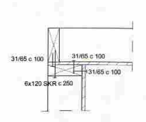
SAMSETNING Á 90° INNHORNI
