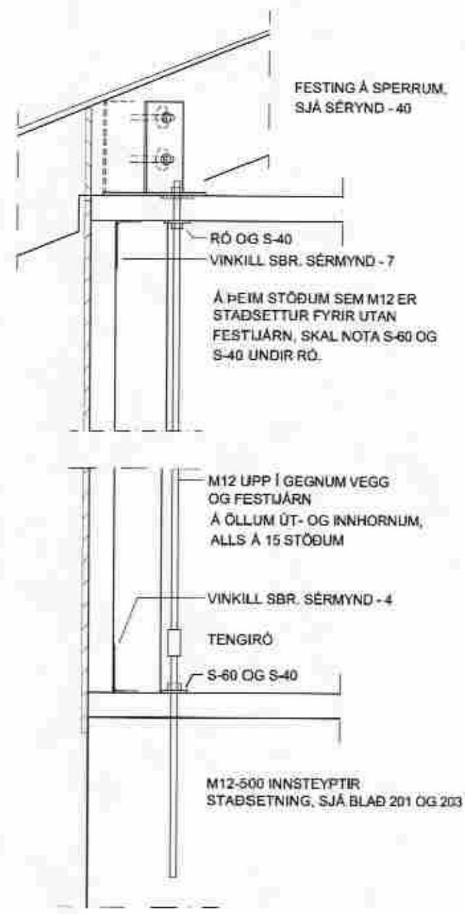
SAMSETNING Á 2- OG 3-FÖLDUM STÖÐUM, 4-FALDAR STÖÐIR BOLTA SAMAN, SJÁ SÉRYMYNDIR 3 OG 13 OG HLIDAMYNDIR
