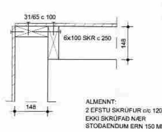
SAMSETNING Á 90° ÚTHORNI
