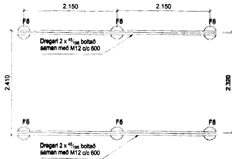
Dregarar og undirstöðusúlar mkv: 1:50
