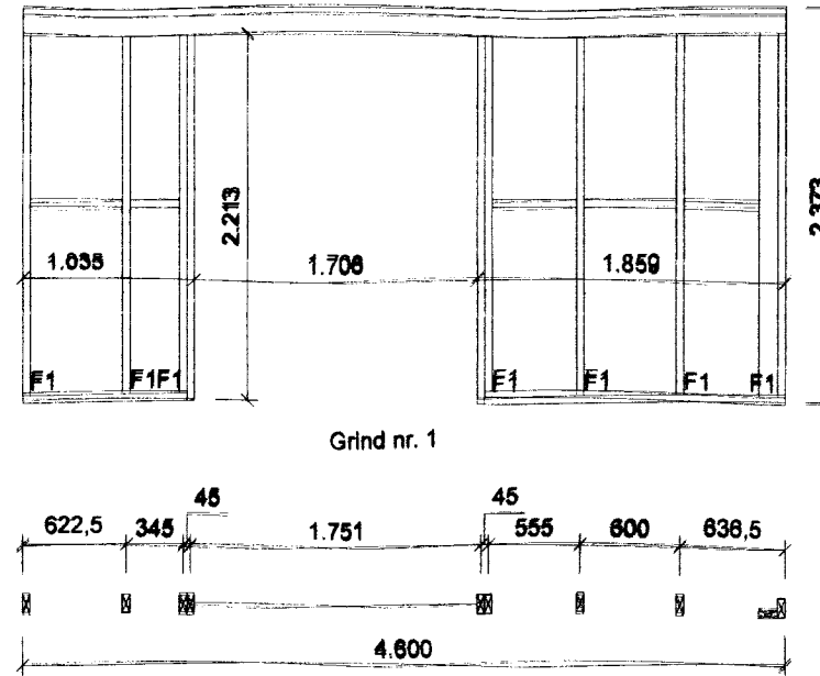
Veggjagrindur mkv: 1:50
