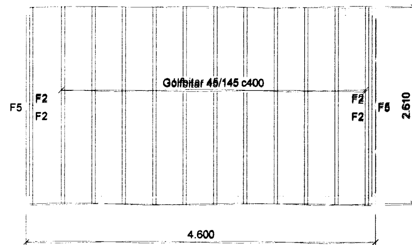
Gólfbitaplan mkv: 1:50
