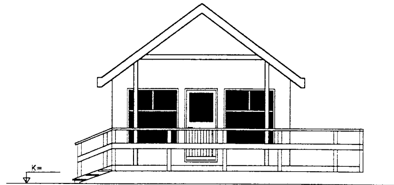
SUÐURHLÍÐ MKV. 1:50
