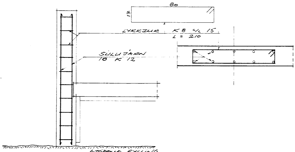
SNID B-B 1:20
