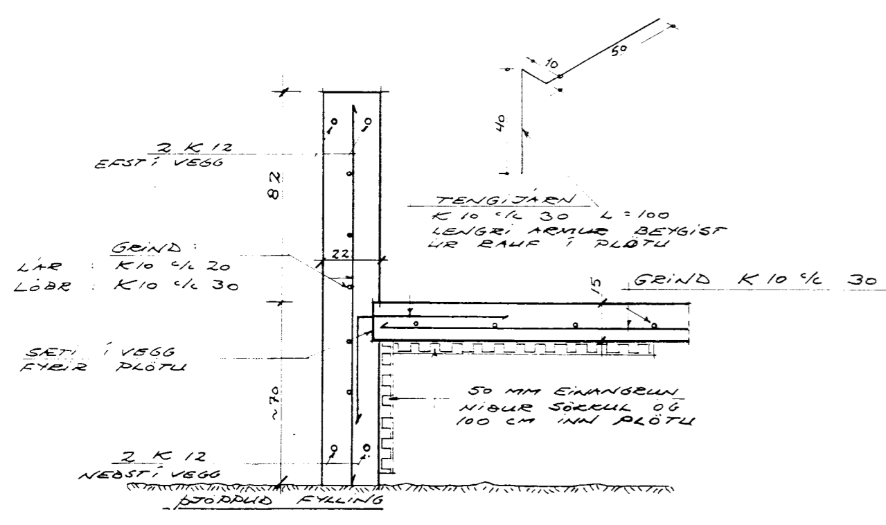
SNID A-A 1:20
