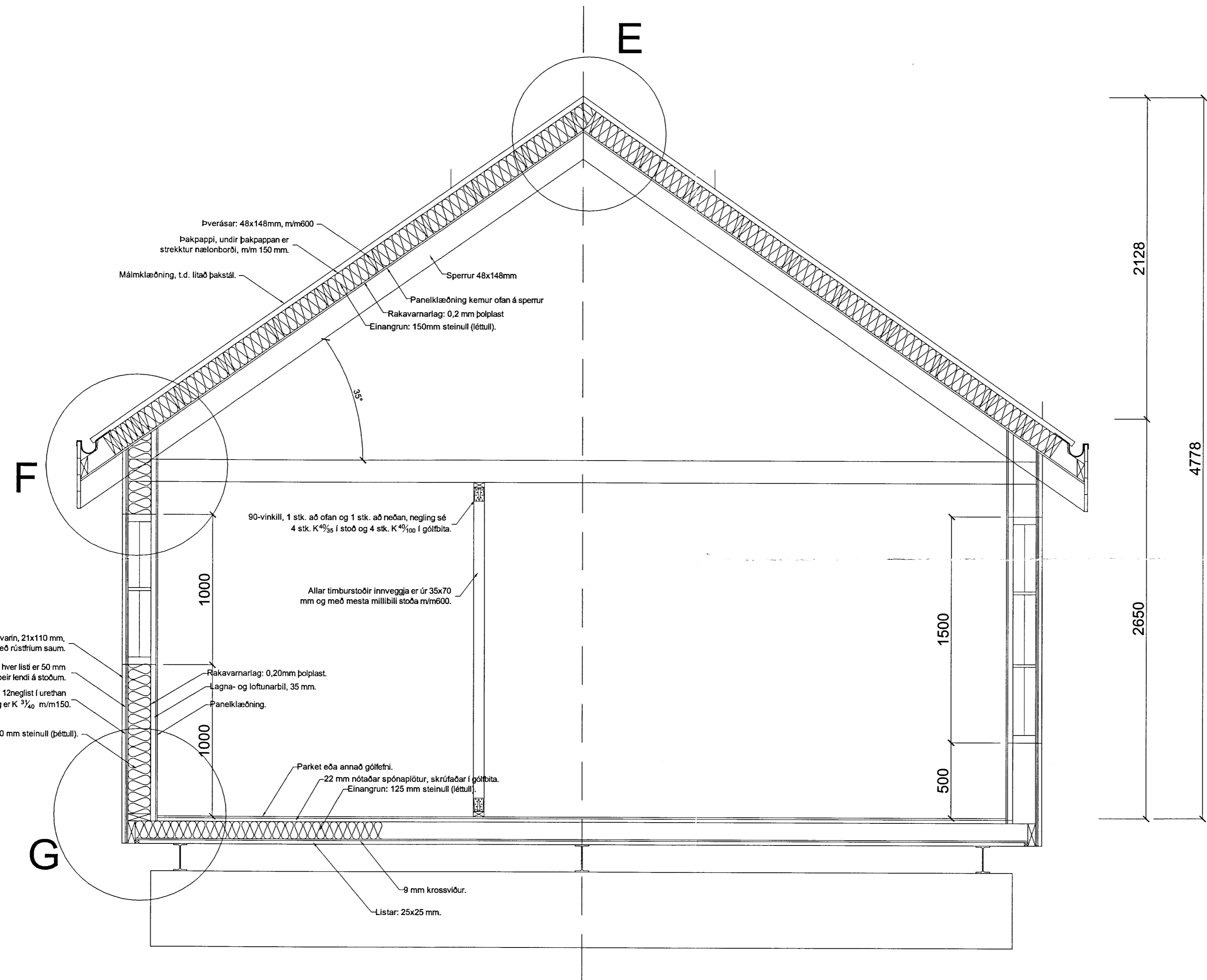
Þversnið í sumarhús með efnisskýringum.
