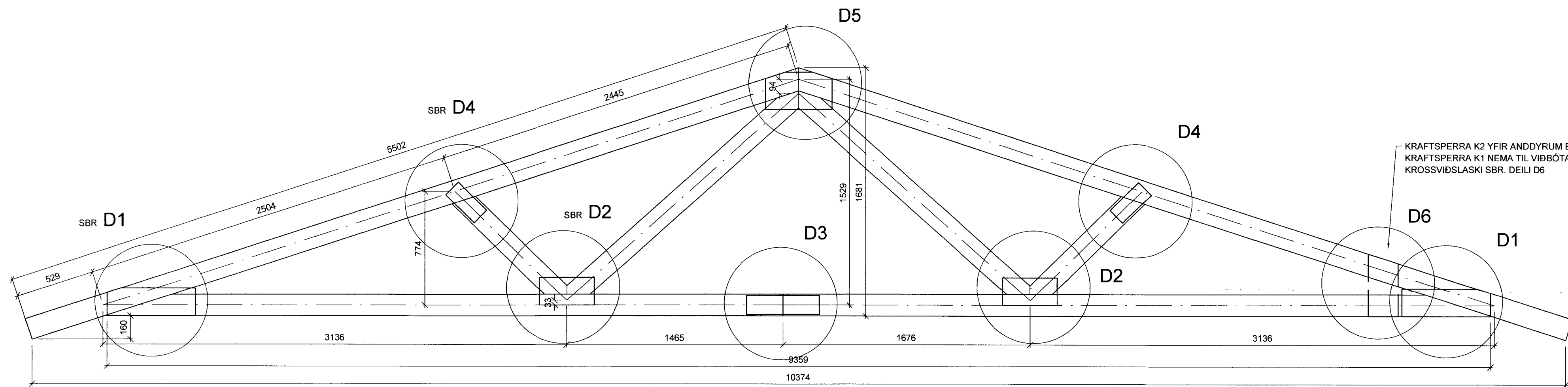
KRAFTSPERRA K1 (K2) 1:20
