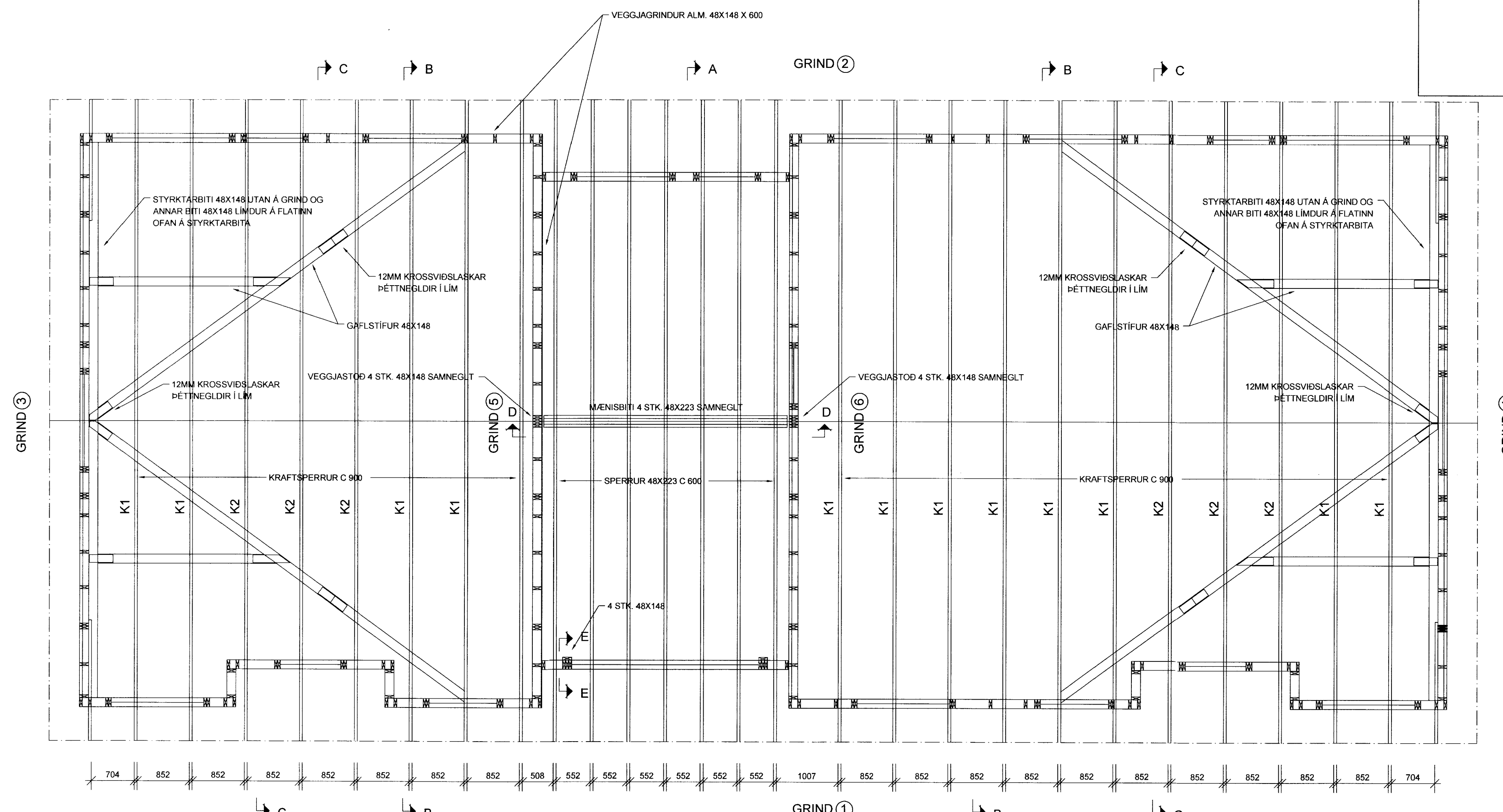
GRUNNMYND ÞAKS 1:50
