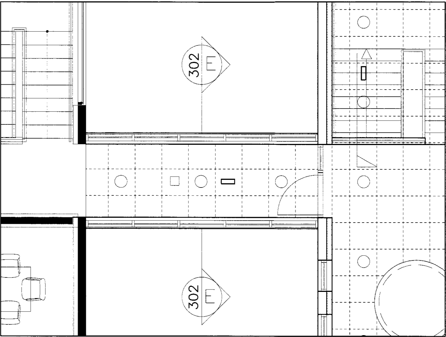
GRUNNMÝND 2.HÆÐ - tengibrú 1:50
