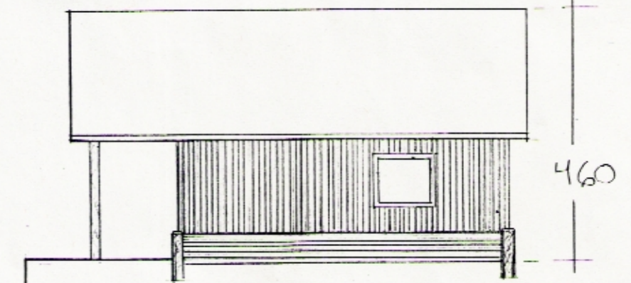
ÖSTUR HLÍÐ 1:100
