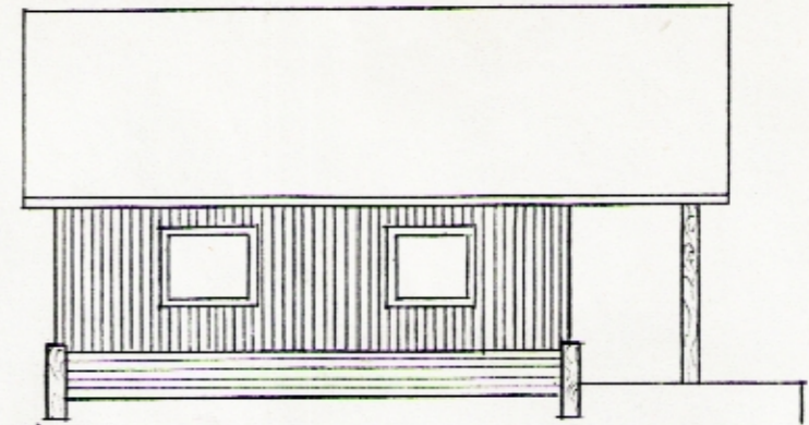
VESTUR HLÍÐ 1:100
