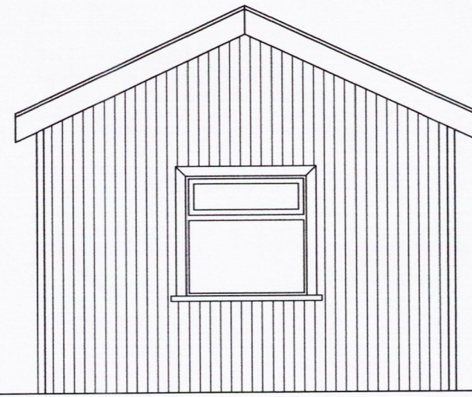
Suður 1:50
