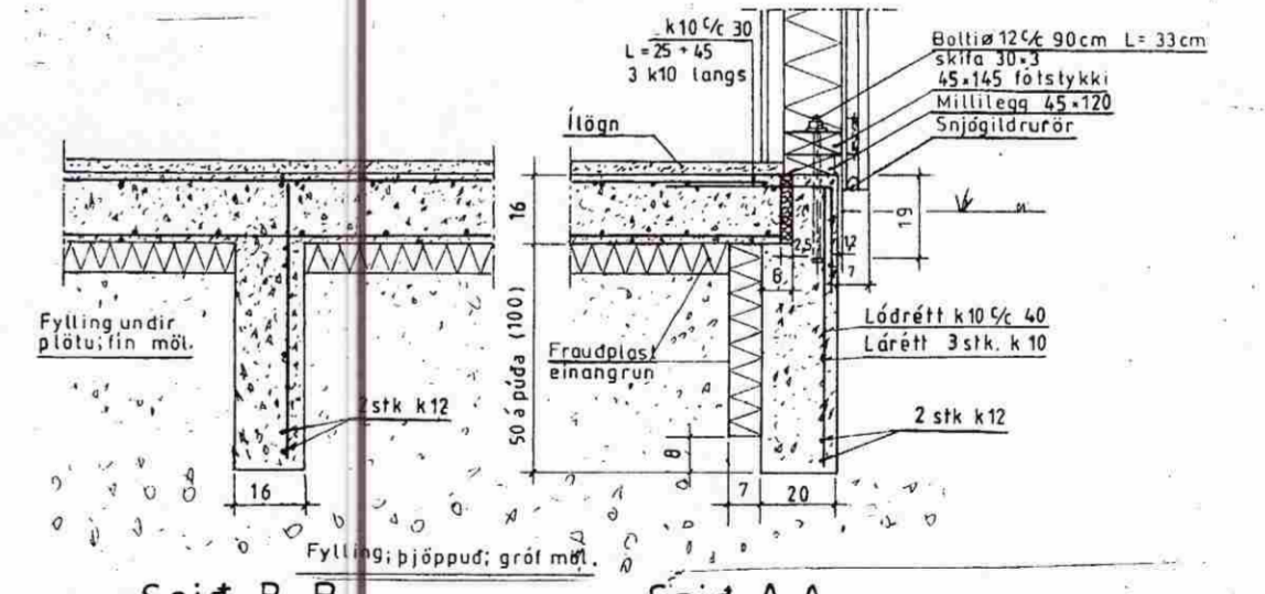
Snid B-B 1:20
