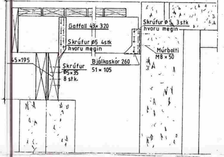
Snid D-D 1:10
