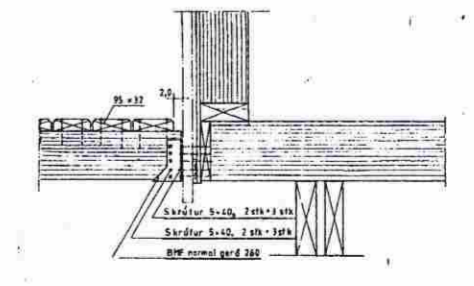
Snid G-G 1:20
