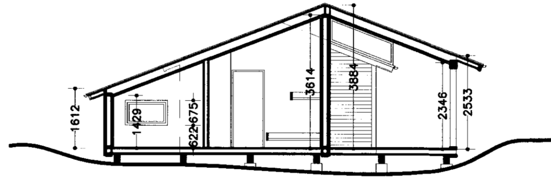
þversnið B-B
